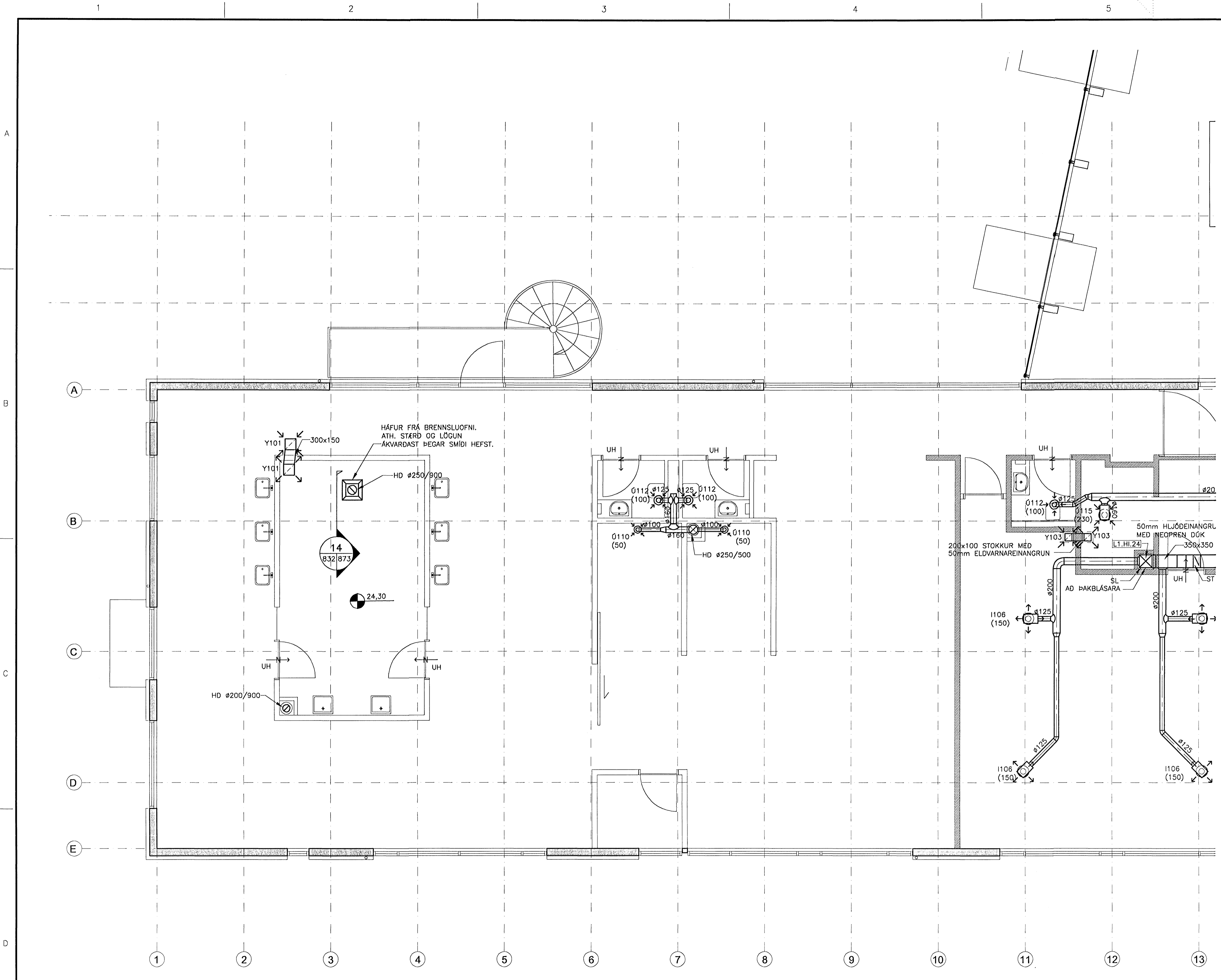
2. HÆÐ, GRUNNMYND MKV. 1
