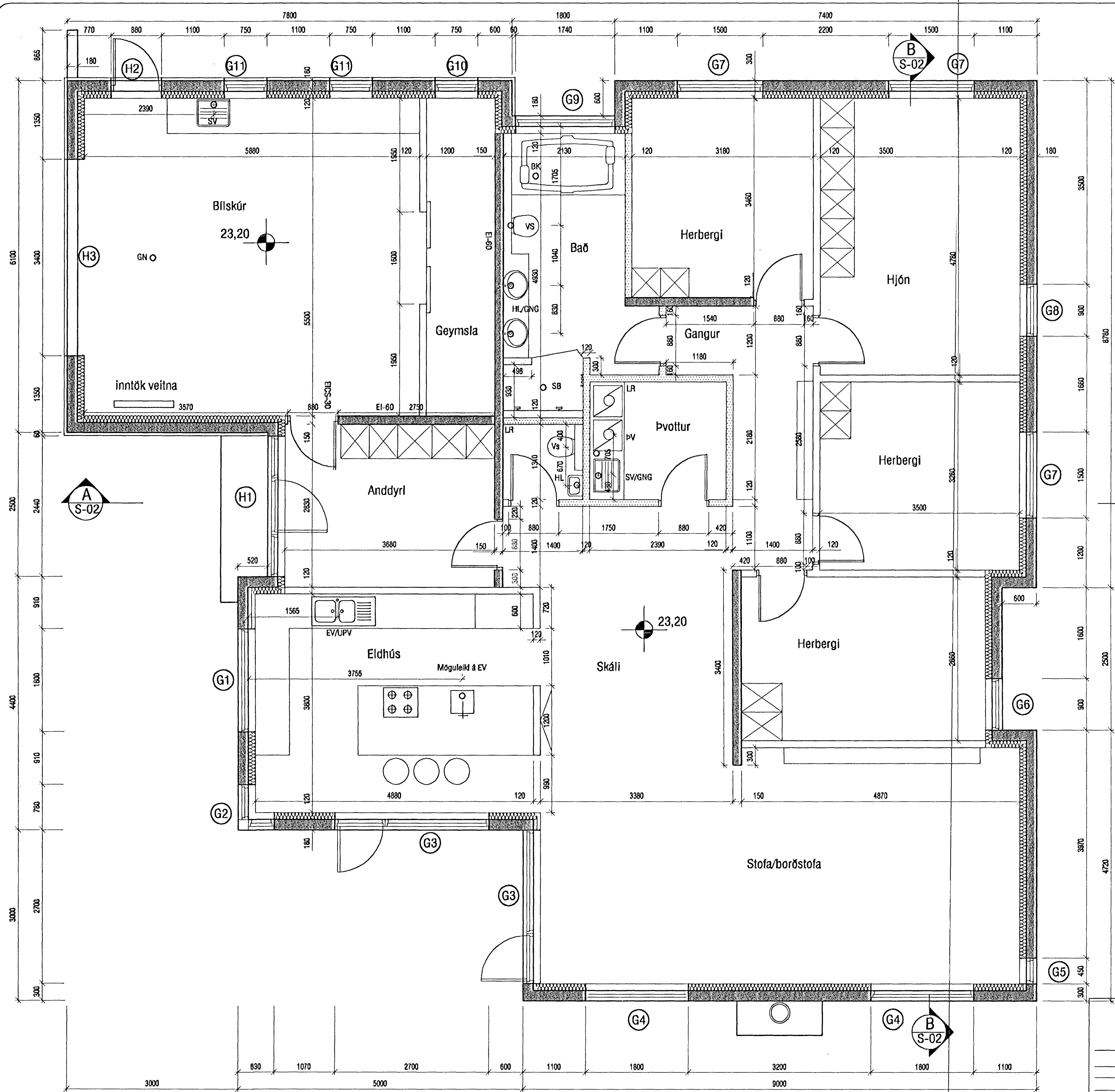
GRUNNMYND 1.HÆÐ
