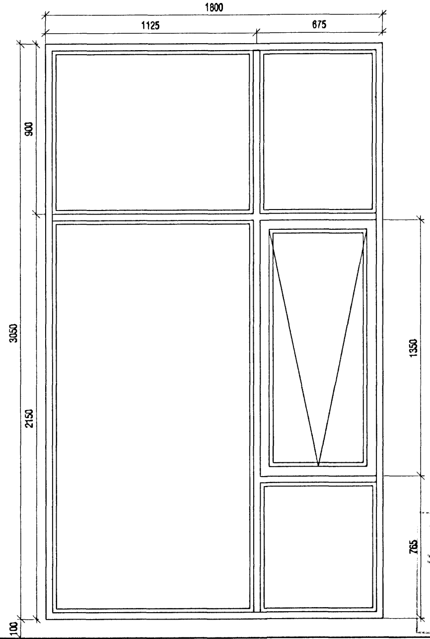
G-4 2 stk (þar af ein spegilmynd)
