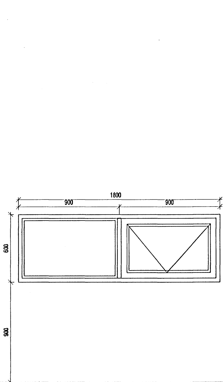
G-1 1 stk
