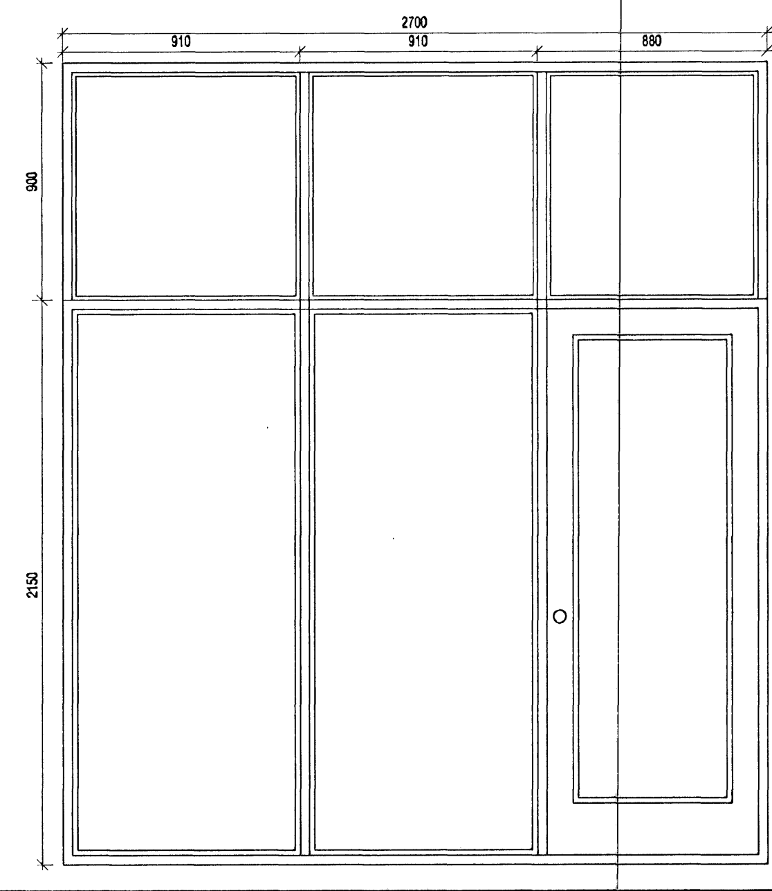
G-3 2 stk (þar af ein spegilmynd) opnun hægri út opnun vinstri út
