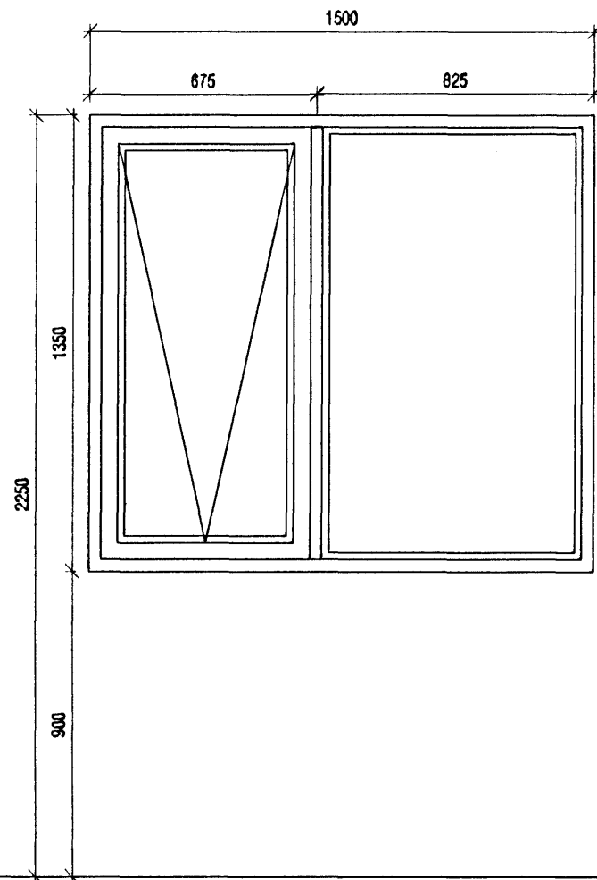
G-7 3 stk. (þar af 1 spegilmynd)
