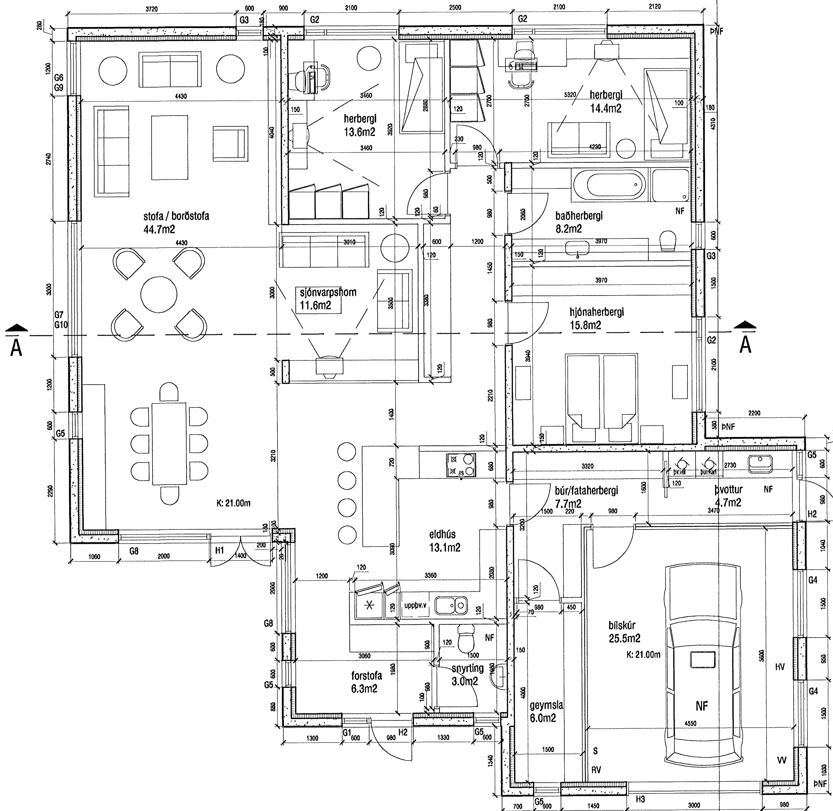
Grunnmynd mkv. 1:50
