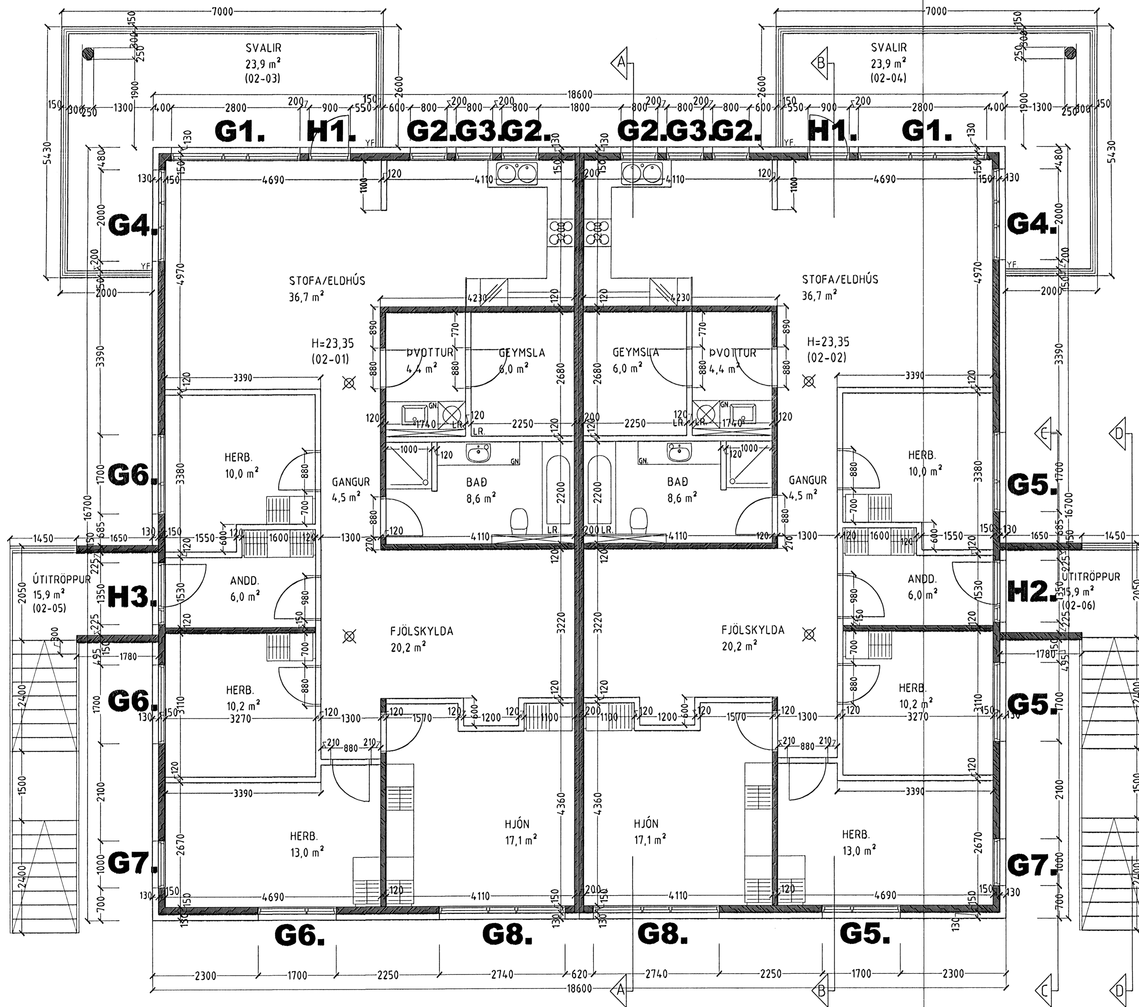
GRUNNMYND 2. HÆÐ MKV. 1:50.
