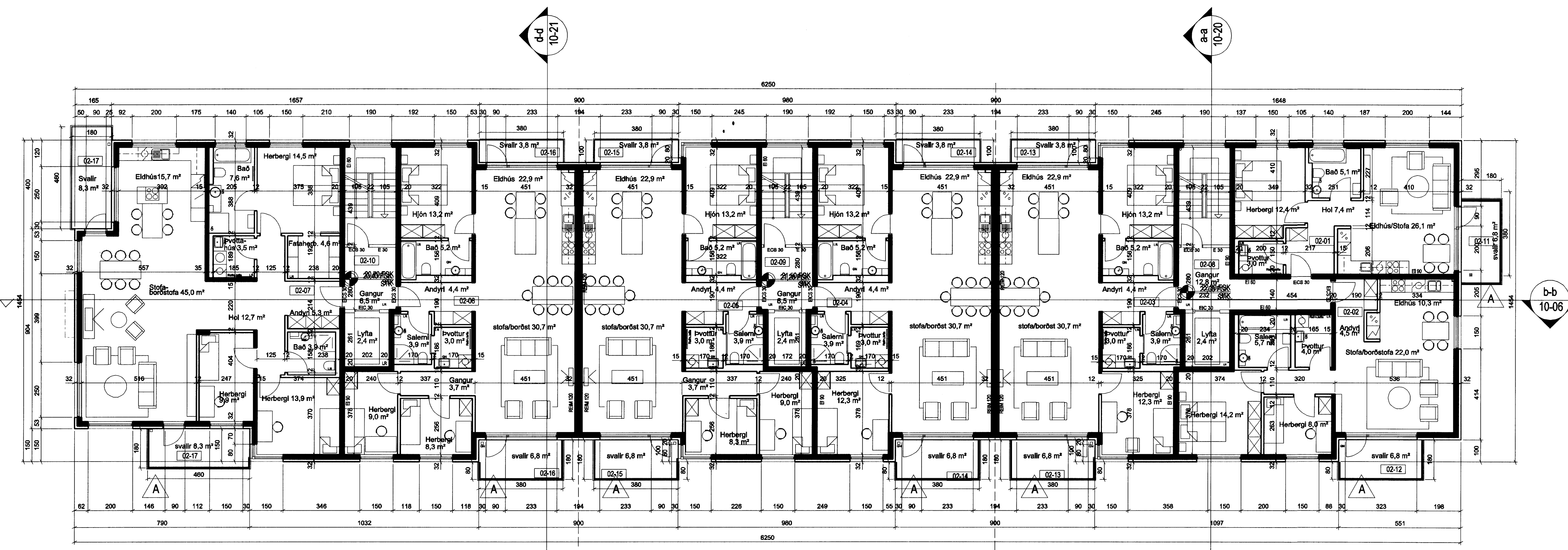
GRUNNMYND 2. HÆÐ 1:100
