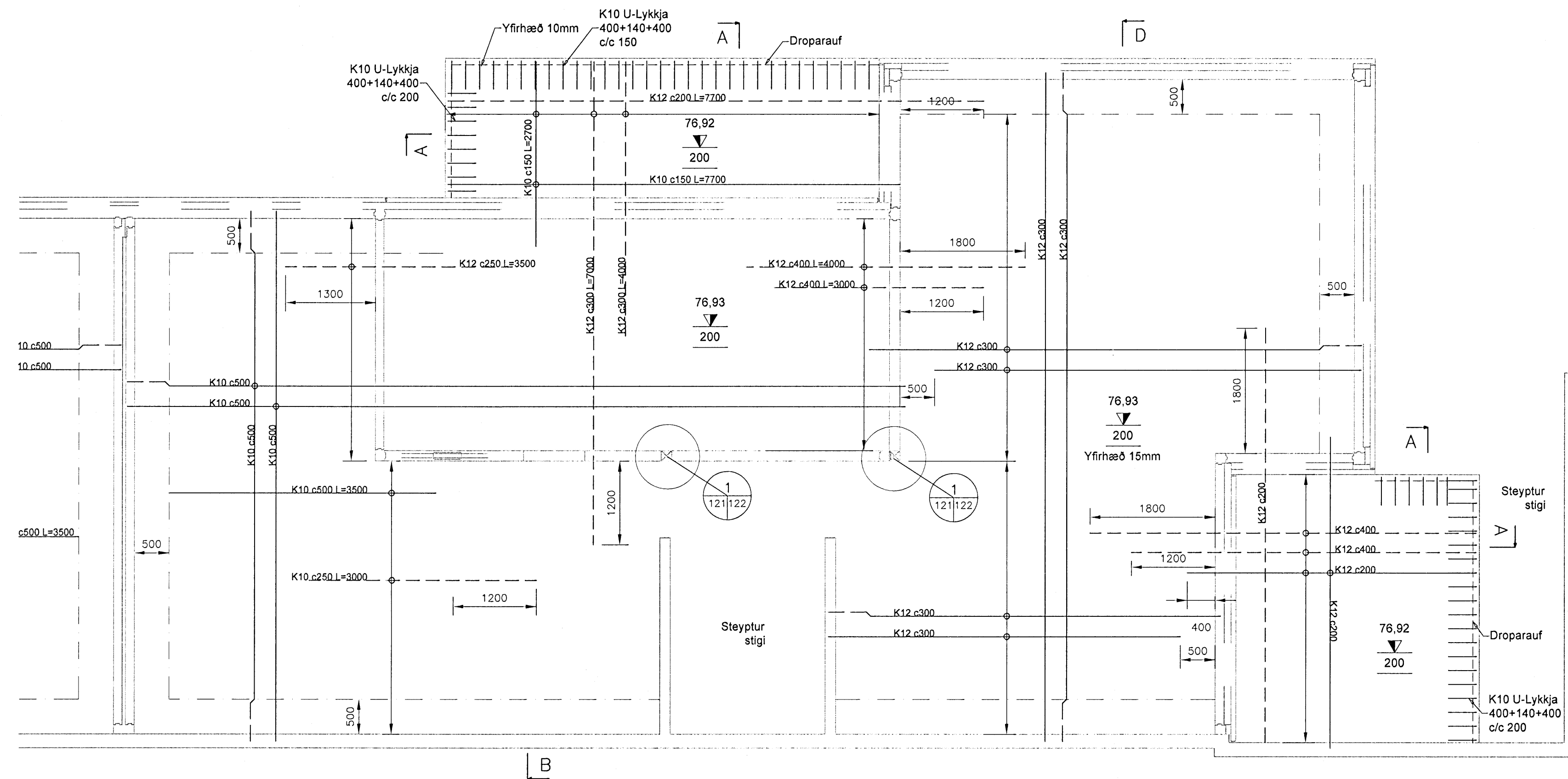
GRUNNMYND 1:50
