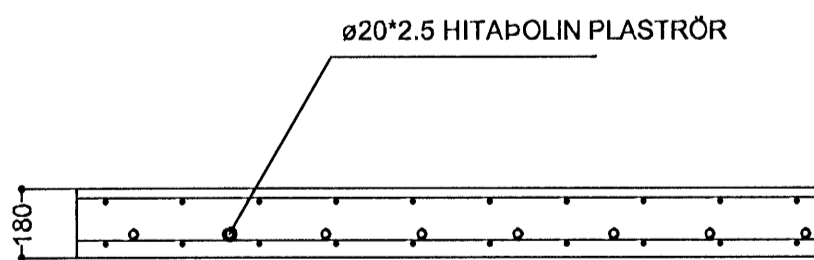
SNEIÐING Í GÓLFPLÖTU mkv. 1:20
