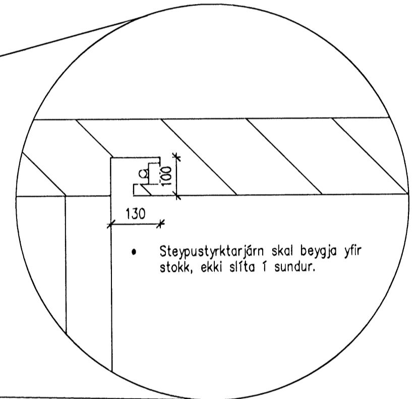
Úrtak fyrir ljósastökk, 1:10
