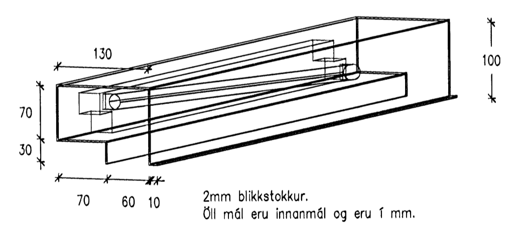
Úrtak fyrir ljósastökk, 1:10
