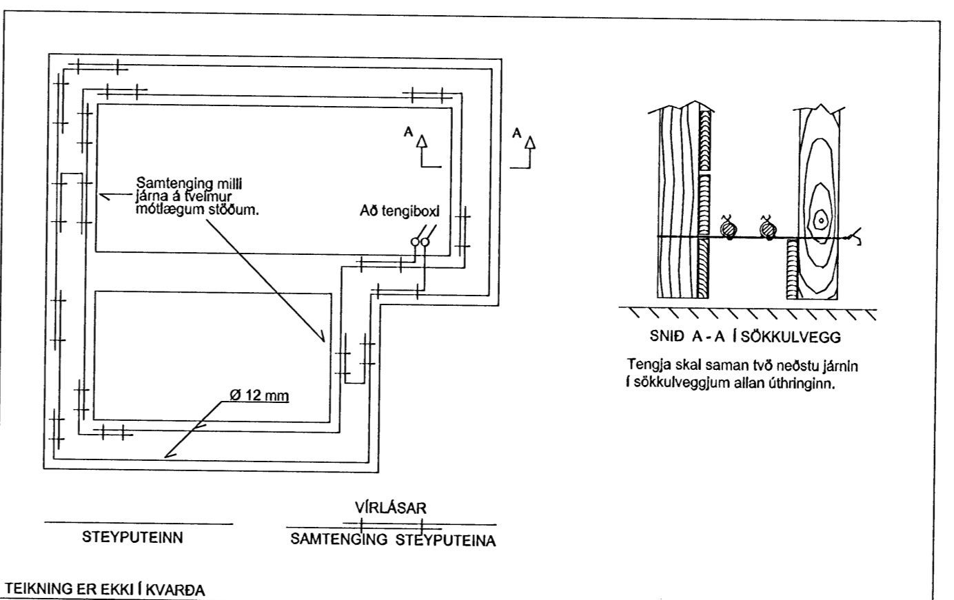
TEIKNING ER EKKI Í KVARÐA FYRIRMYND GRUNNMYND SÖKKULVEGGJA DÆMIGERÐUR FRÁGANGUR
