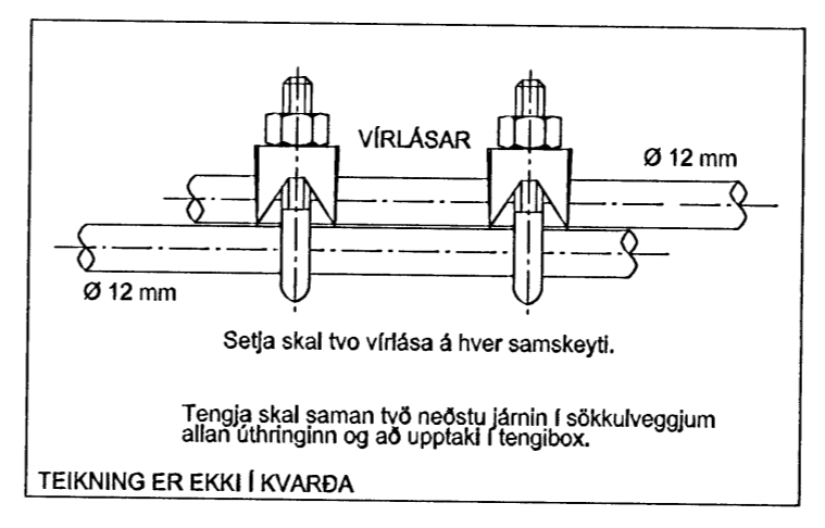
TEIKNING ER EKKI Í KVARÐA SAMTENGING STEYPUPEINA DÆMIGERÐUR FRÁGANGUR
