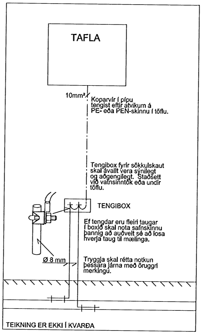
TEIKNING ER EKKI Í KVARÐA SNID Í TÖFLUVEGG DÆMIGERÐUR FRÁGANGUR
