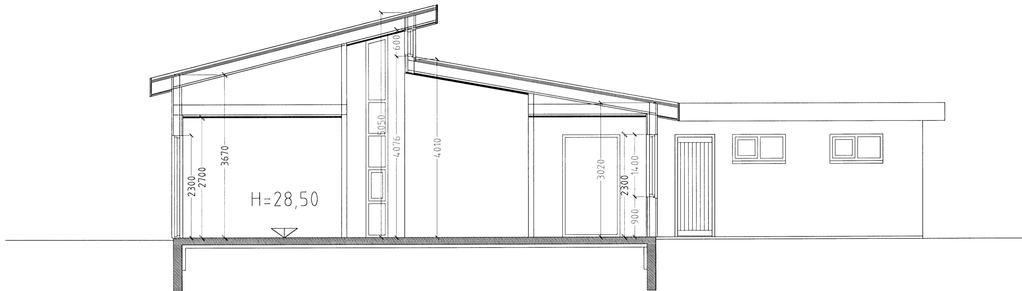
SNIÐMYND A-A MKV. 1:50.
