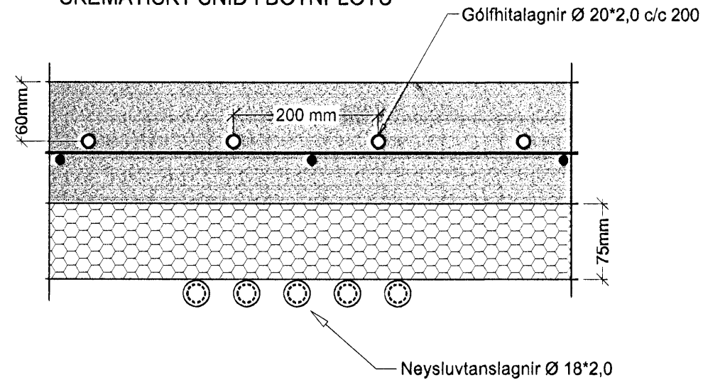
SKEMATISKT SNID Í BOTNPLÖTU
