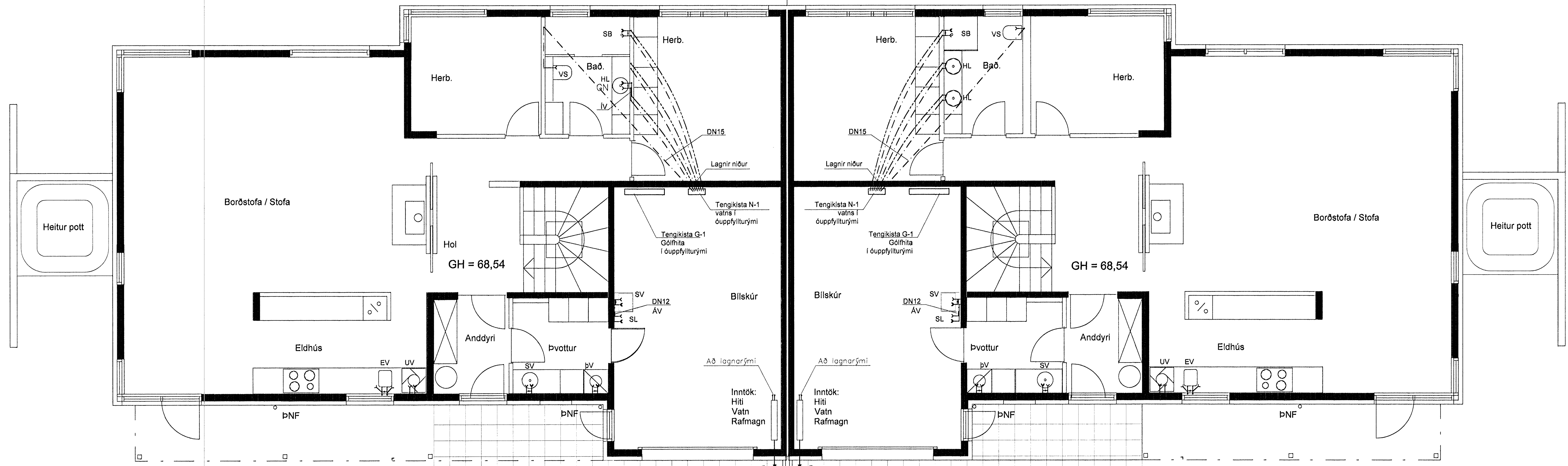
Grunnmynd húsnr.10 1 = 50 mm
