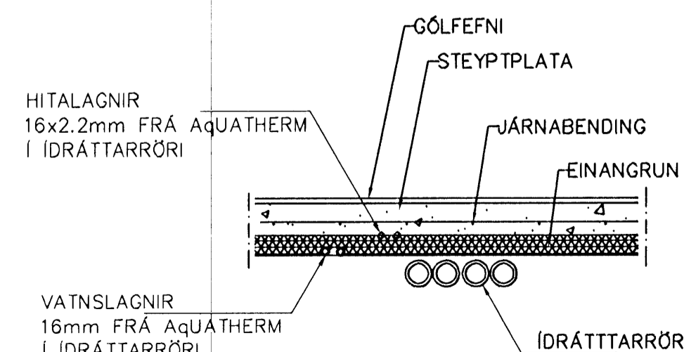
LAGNIR, SNIÐ, 1:20
