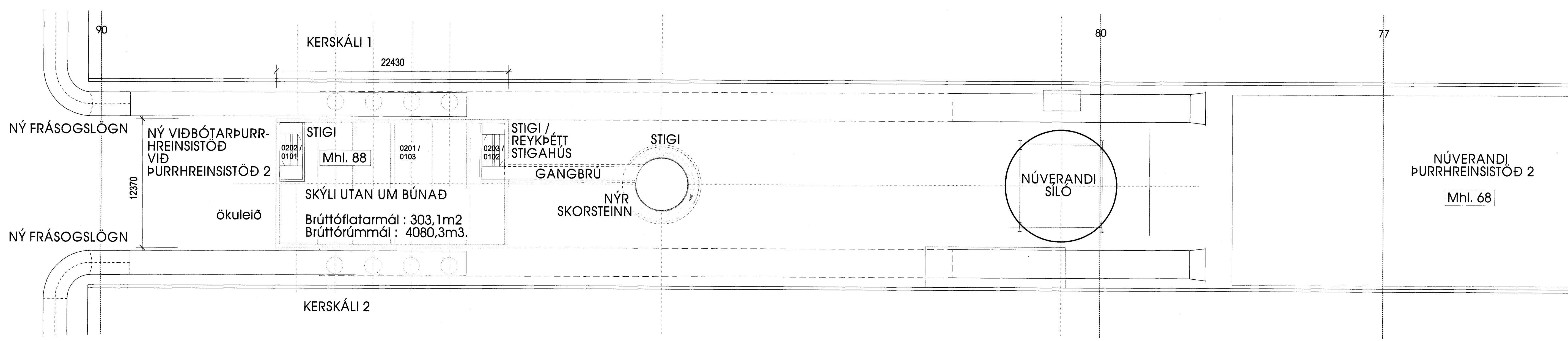
1 ÞAKMYND / GRUNNMYND ÞURRHREINSISTÖÐ 2 mkv. 1:200
