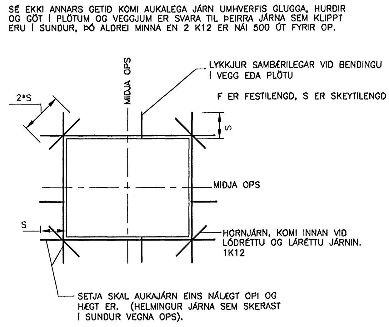
D11 ALMENNUR FRÁGANGUR JÁRNA Í KRINGUM OP
