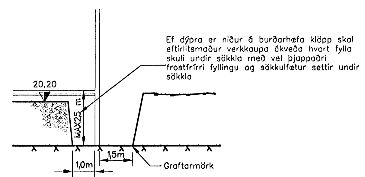
DÆMIGERT SNID SEM SÝNIR HÁMARKSHÆÐ SÖKKLA 1:100
