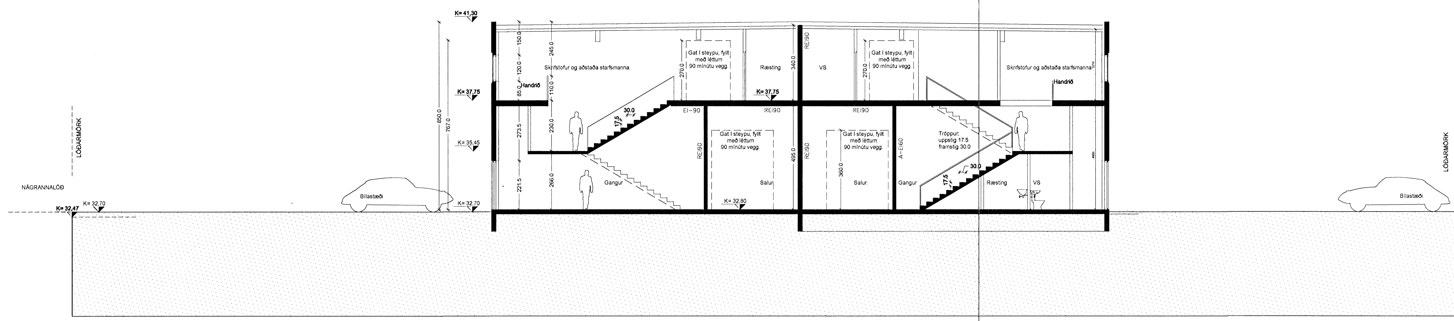
SNÍÐ B-B 1:100
