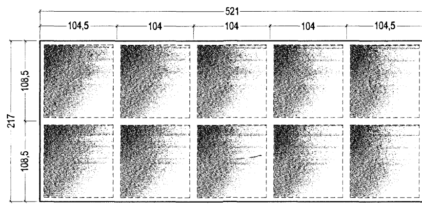
Þakgluggi
