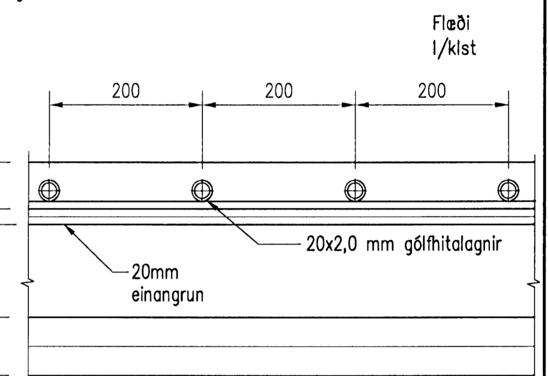
SNÍÐ Í GÓLFHITA 1:5
