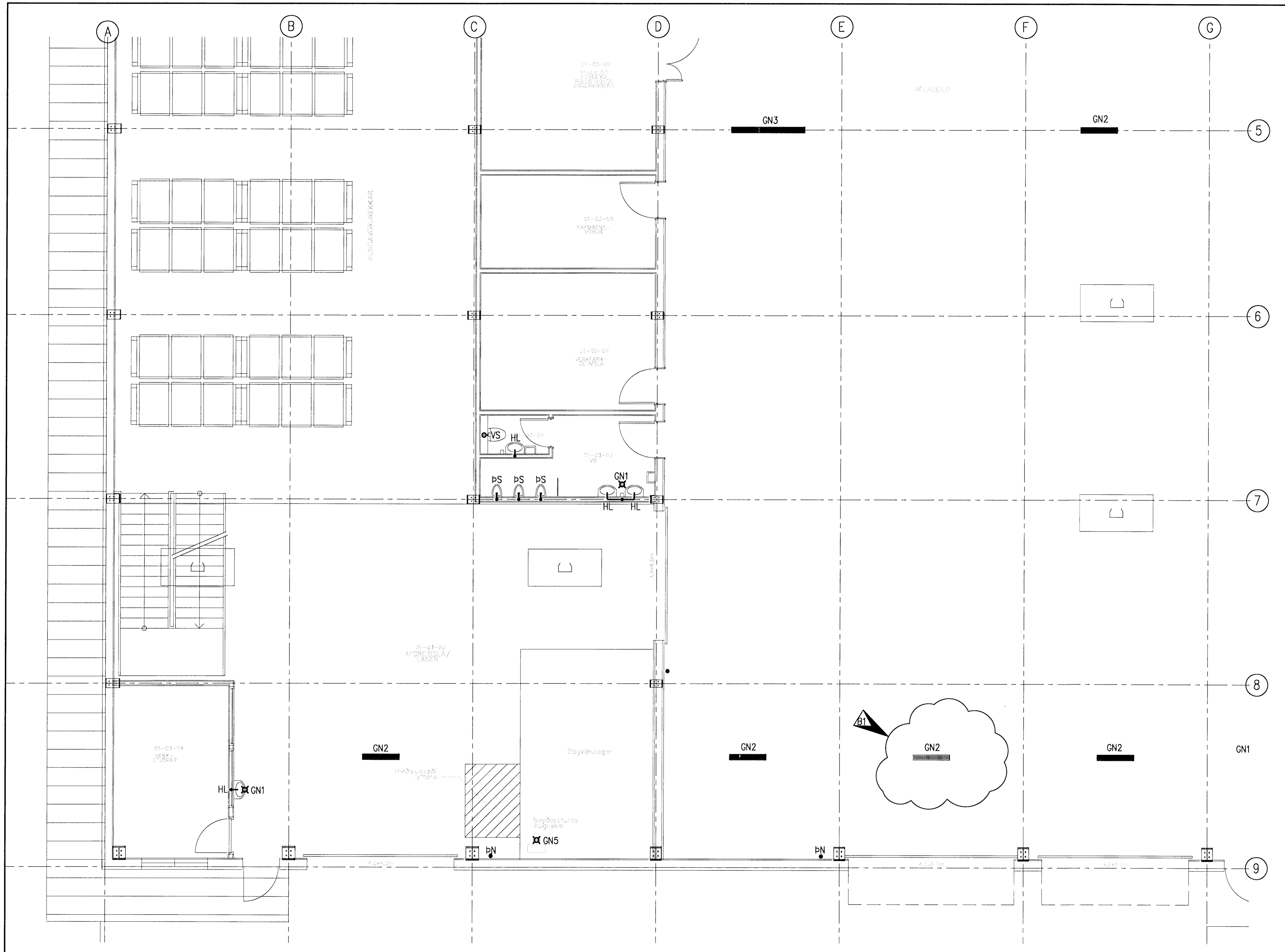
LAGNIR 1. HÆÐ 1:50
