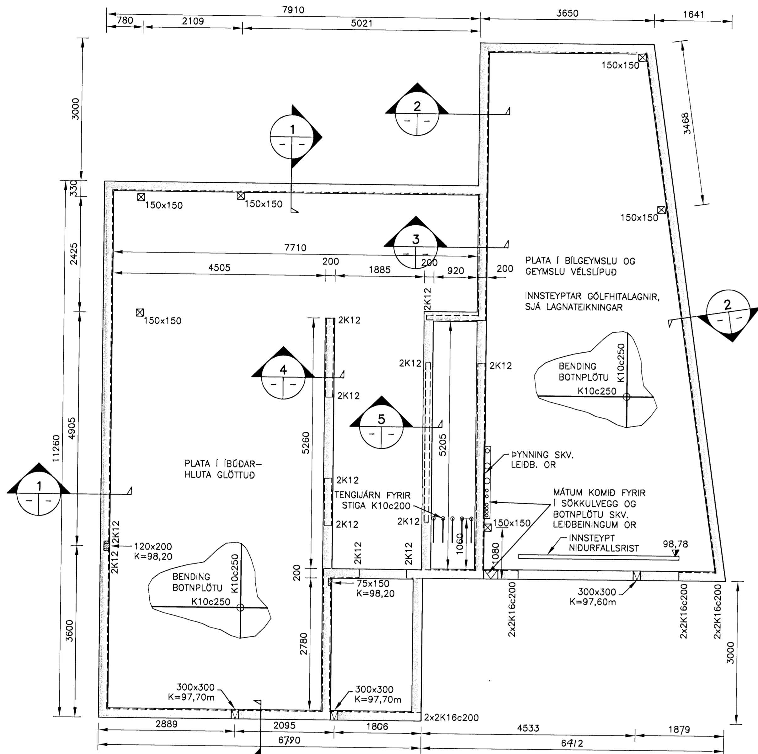
GRUNNMYND MKV. 1
