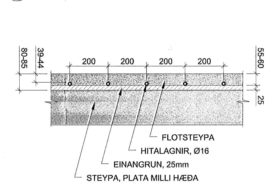
SM2 GÓLFHITALAGNIR 2. HÆÐ 1:10 DÆMIGERT ÞVERSNIÐ
