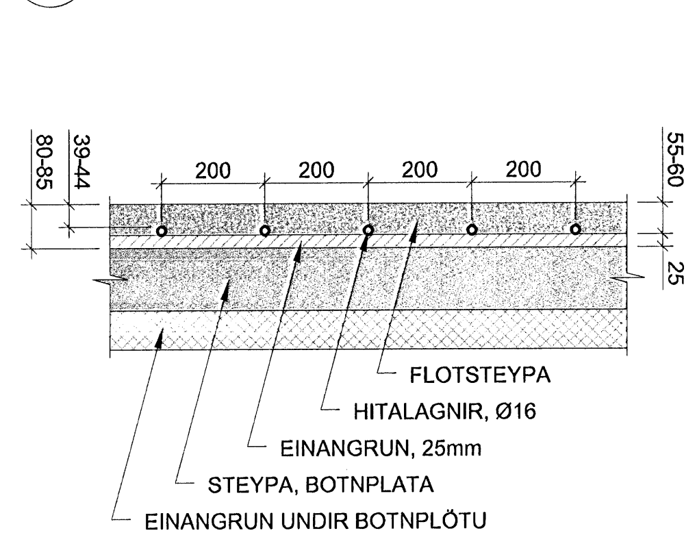
SM1 GÓLFHITALAGNIR 1. HÆÐ 1:10 DÆMIGERT ÞVERSNIÐ
