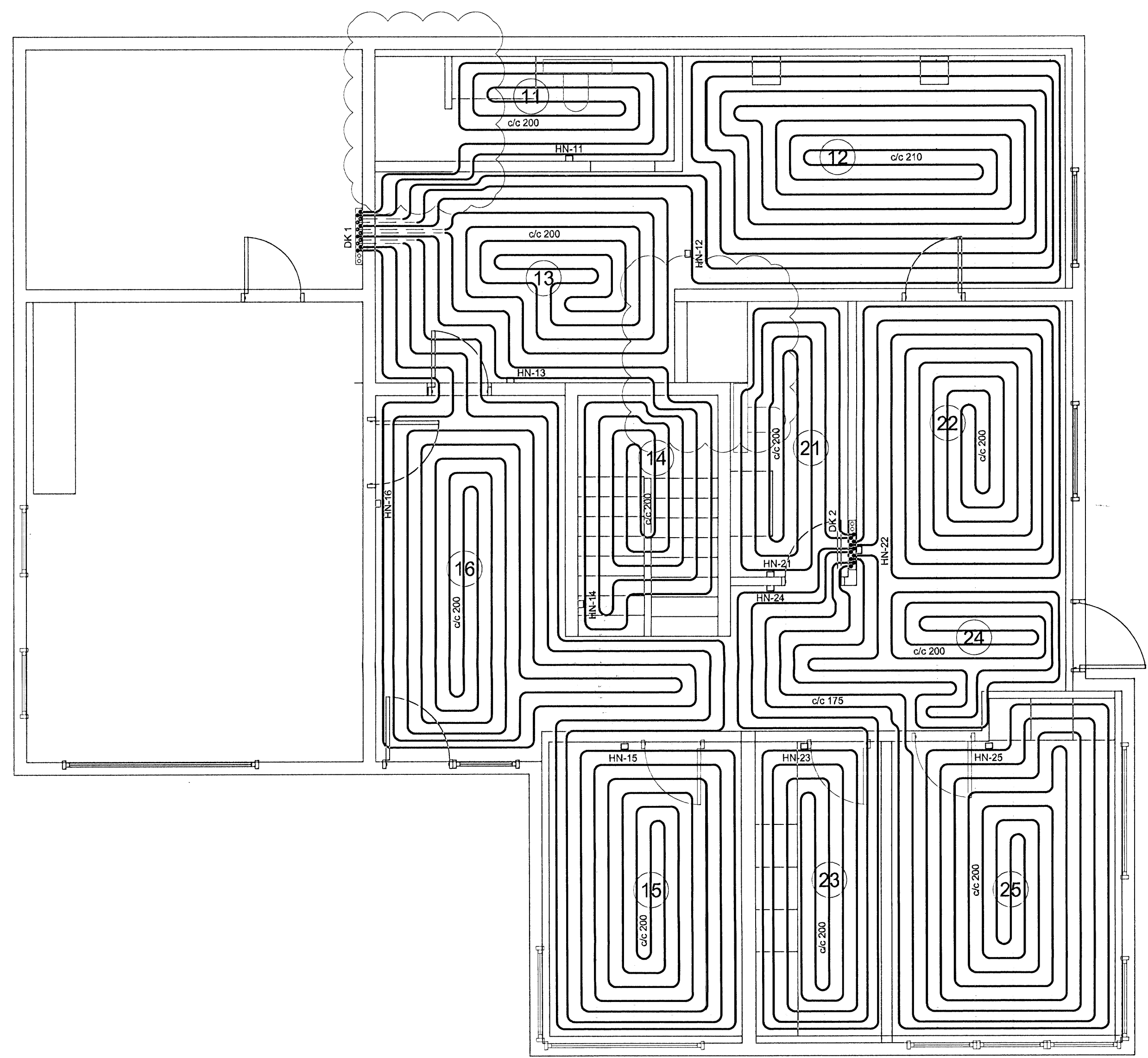
GRUNNMYND - 1. HÆÐ
