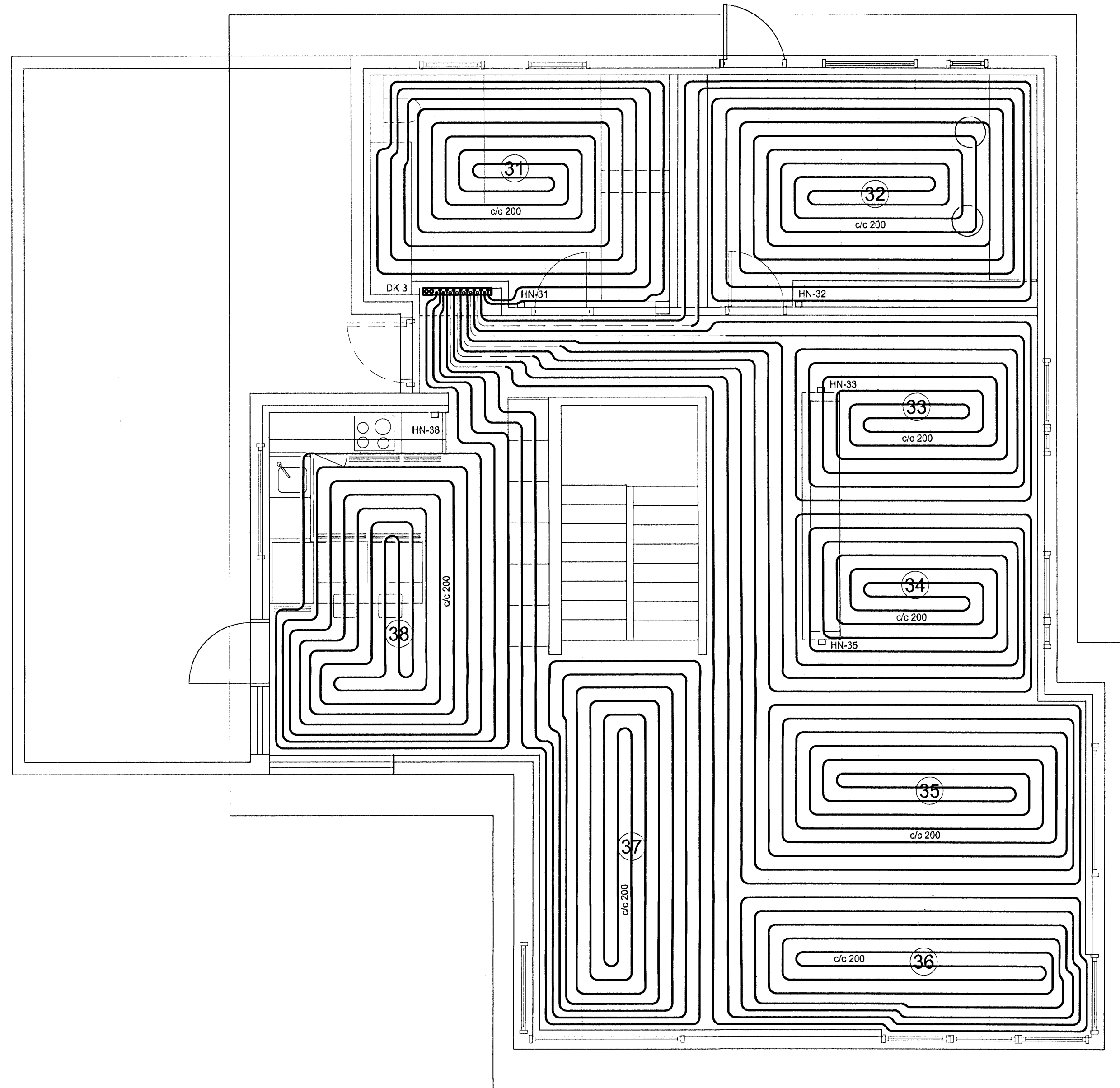
GRUNNMYND - 2. HÆÐ
