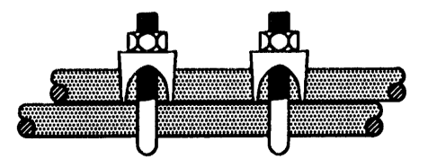
FRÁGANUR Á SAMTENGINGUM STEYPUTEINA FYRIR SÖKKULJARÐSKAUT
