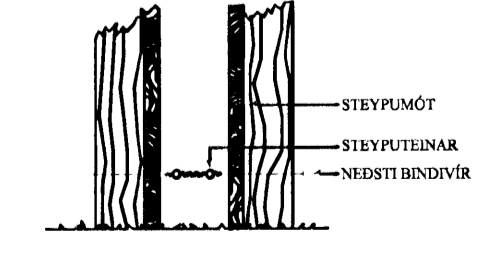
FRÁGANUR Á SAMTENGINGUM STEYPUTEINA FYRIR SÖKKULJARÐSKAUT
