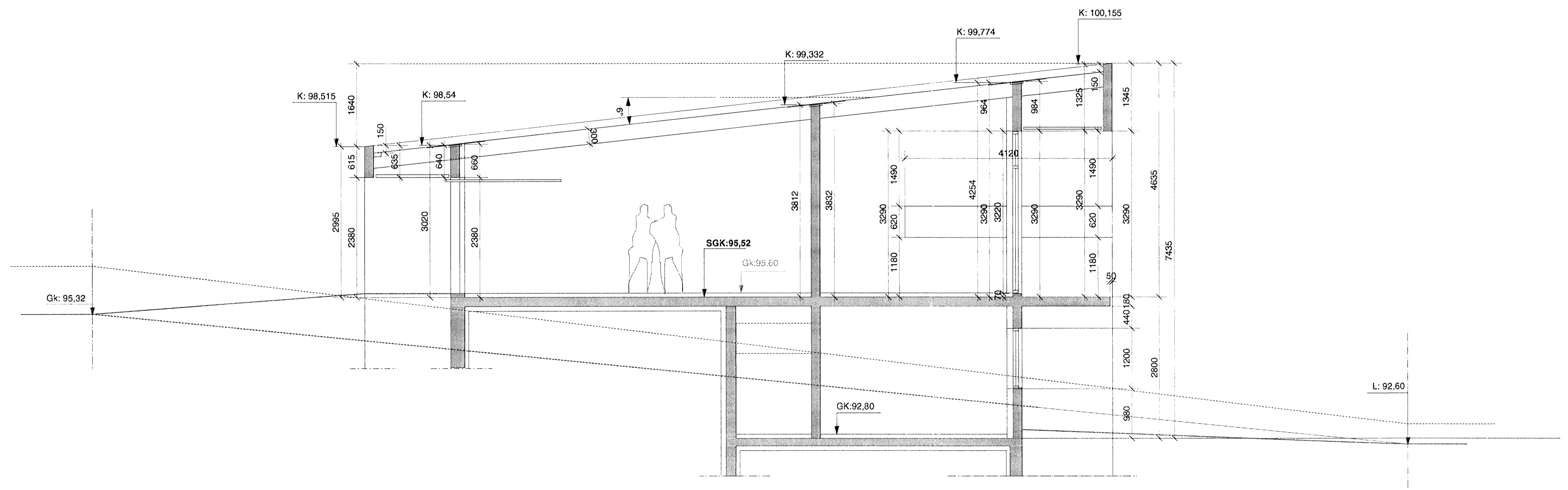
SNIÐ B-B
