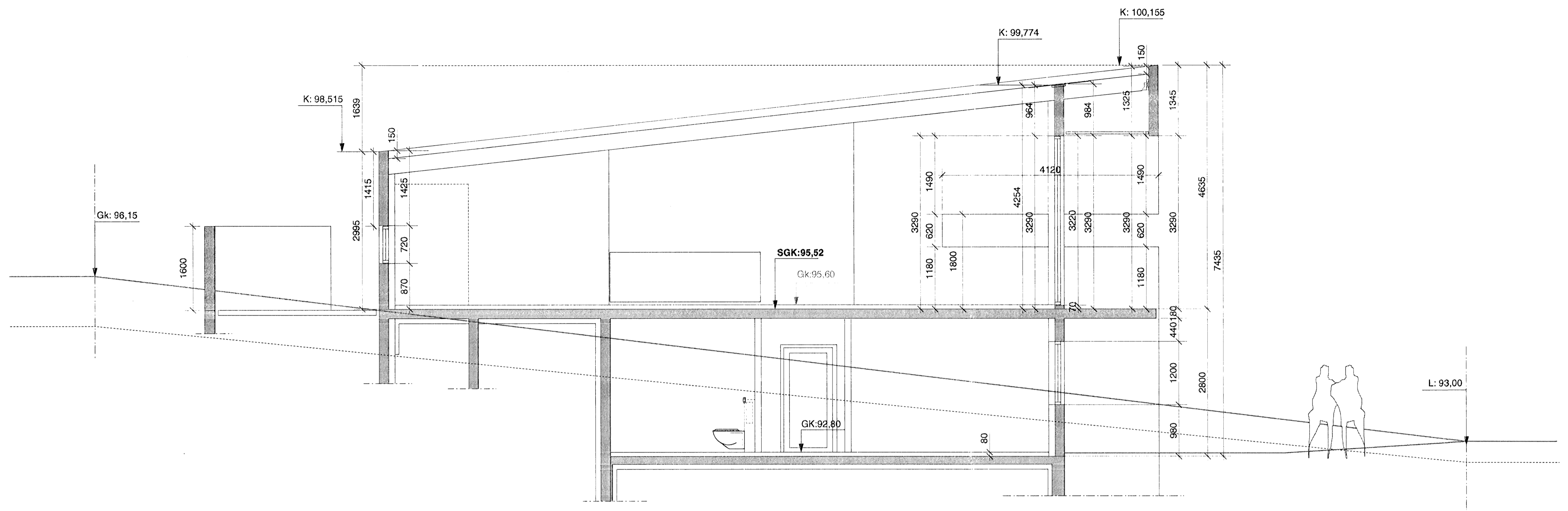
SNIÐ A-A
