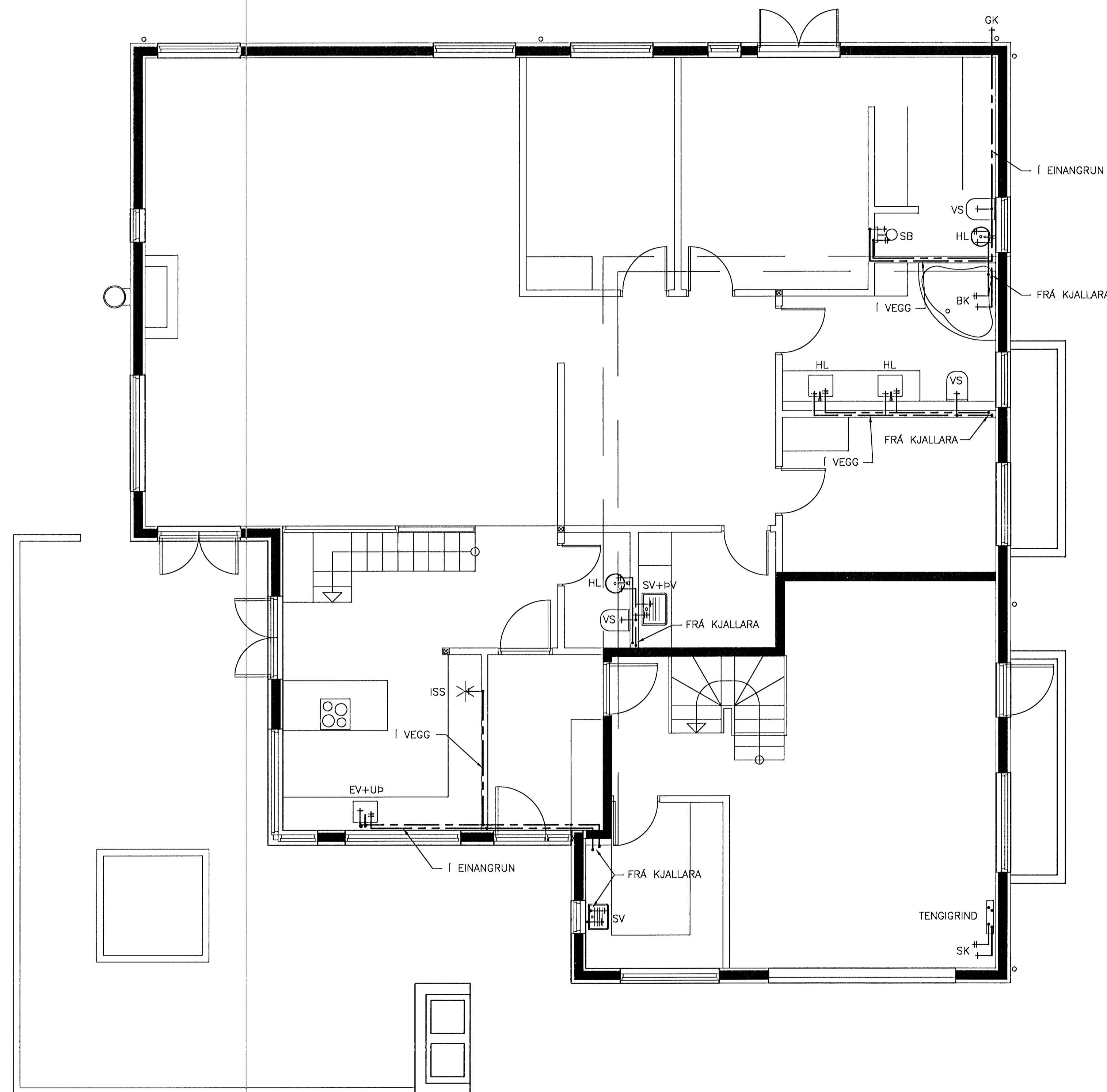
GRUNNMYND 1.HÆÐ. 1:50
