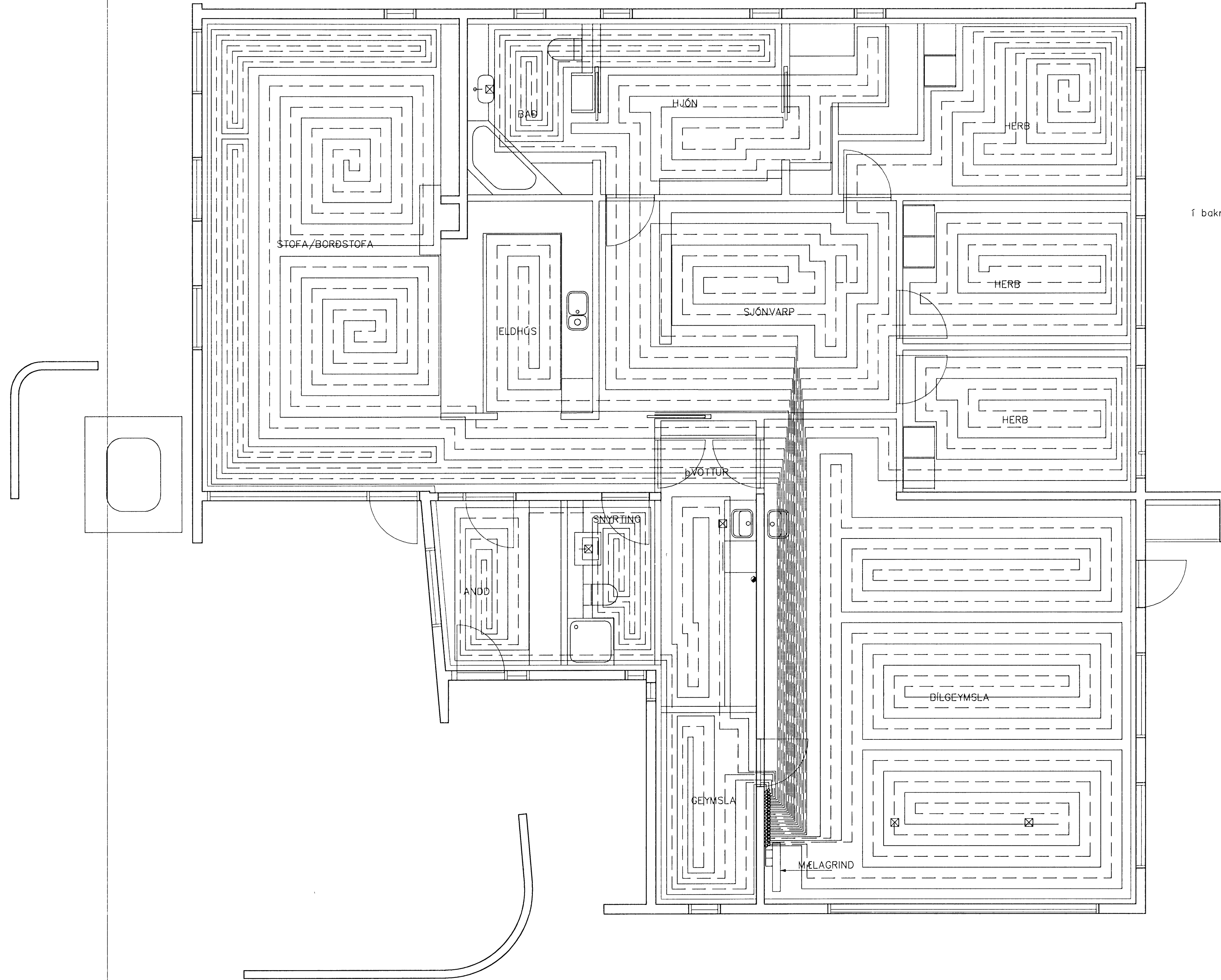
GRUNNMYND 1:50
