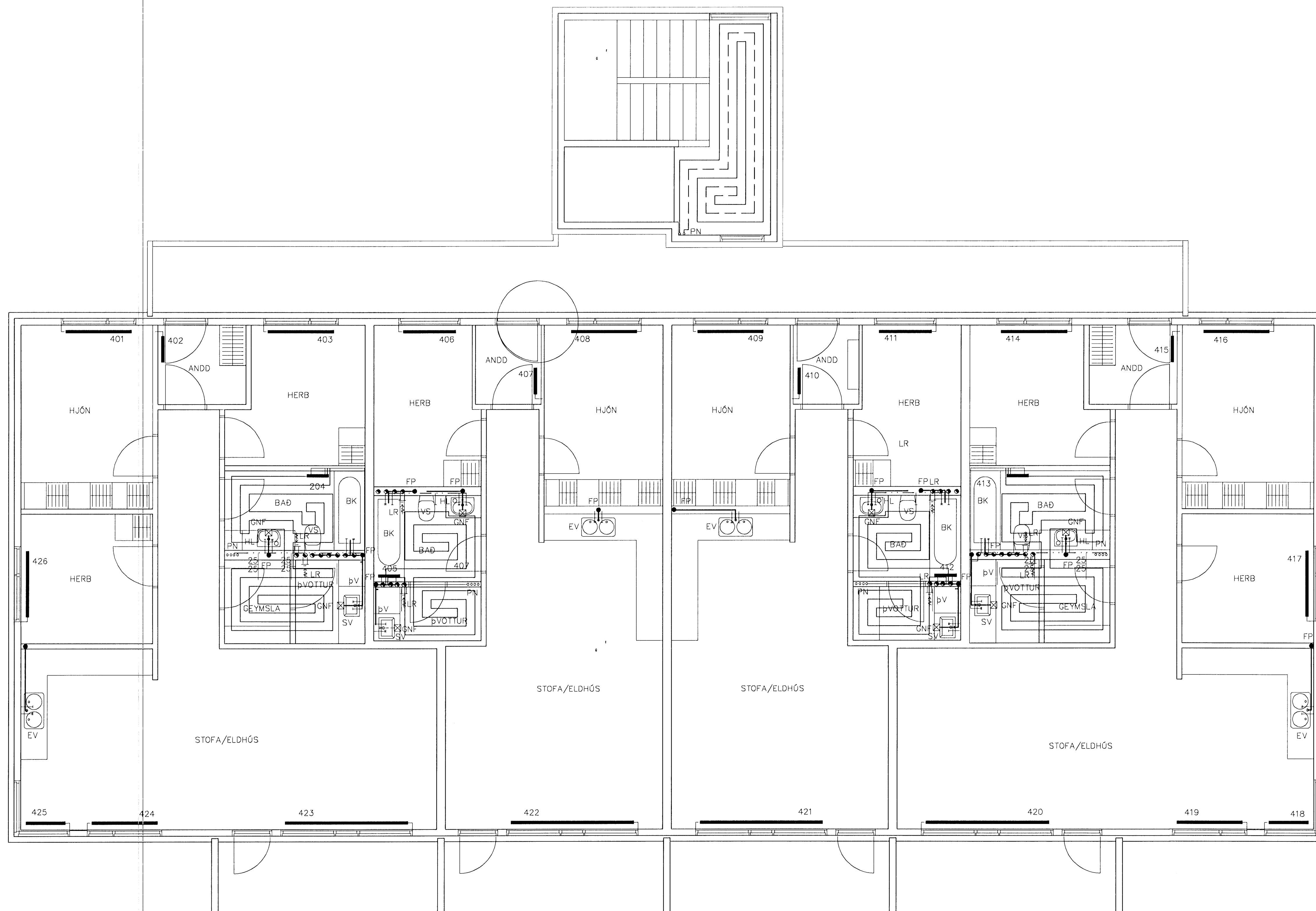
GRUNNMYND 4 HÆÐAR 1:50
