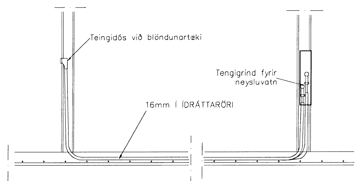
TENGING NEYSLUVATNSLAGNA 1:20
