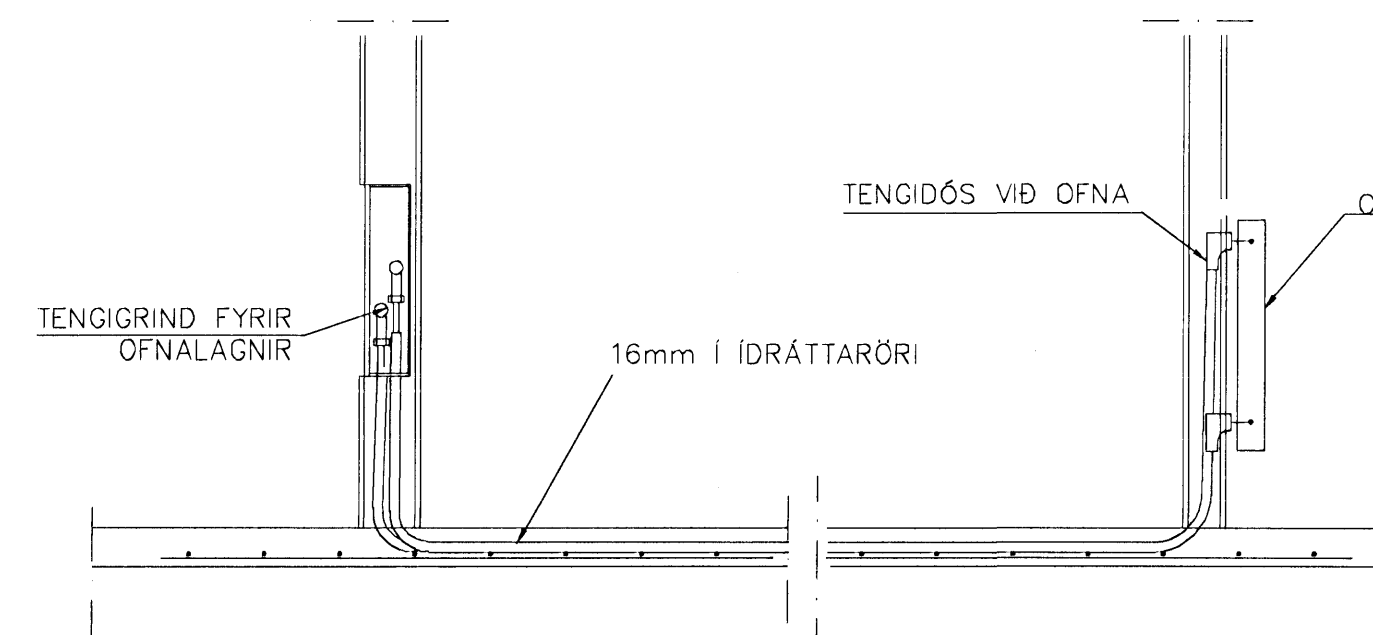
TENGING OFNALAGNALAGNA 1:20
