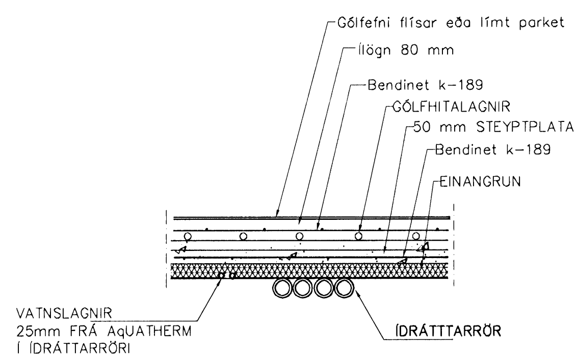
LAGNIR, SNÍÐ Í ÍBÚÐIR, 1:20
