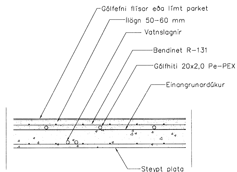
LAGNIR, SNIÐ, 1:20
