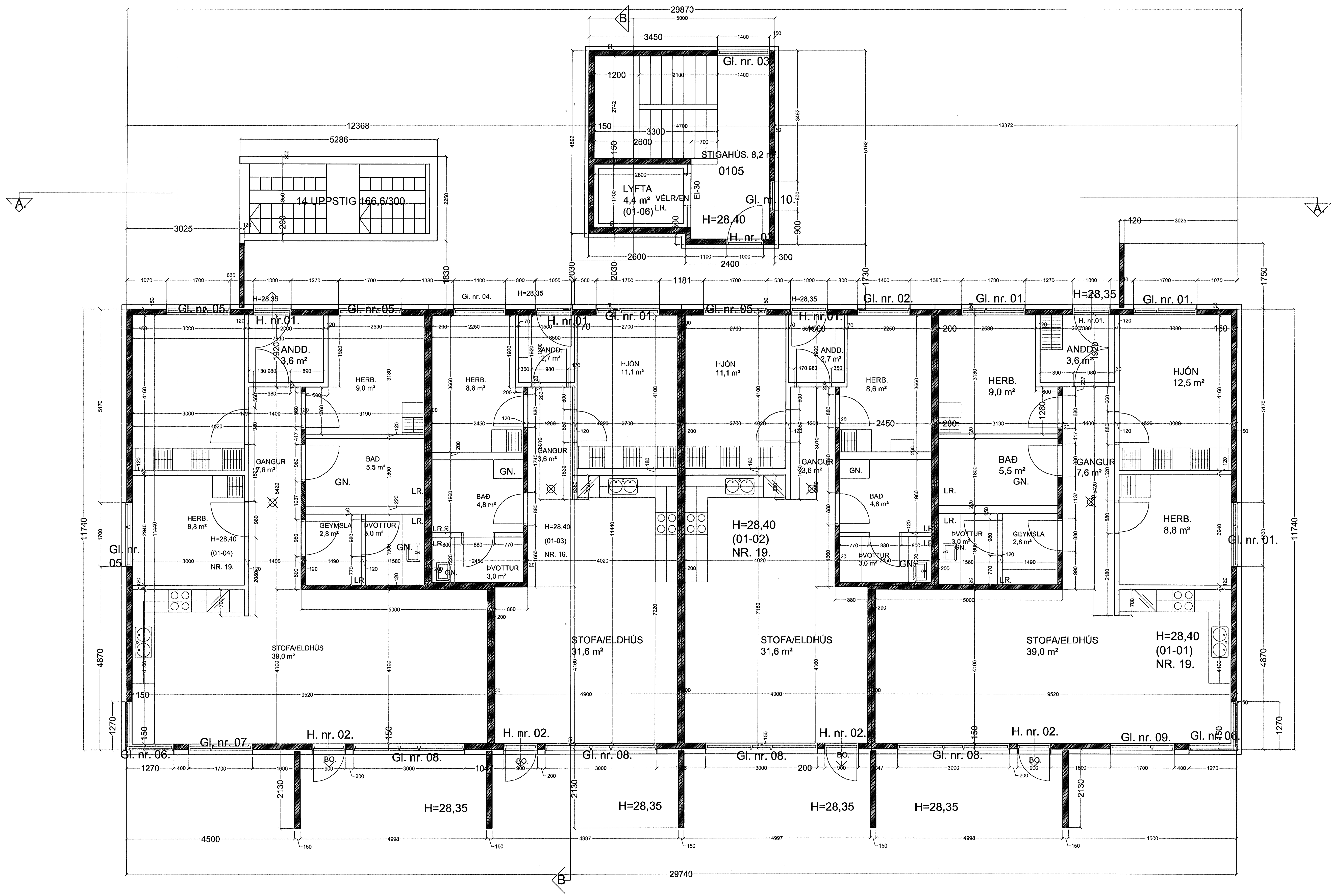
GRUNNMYND 1 HÆÐ. MKV. 1:50.
