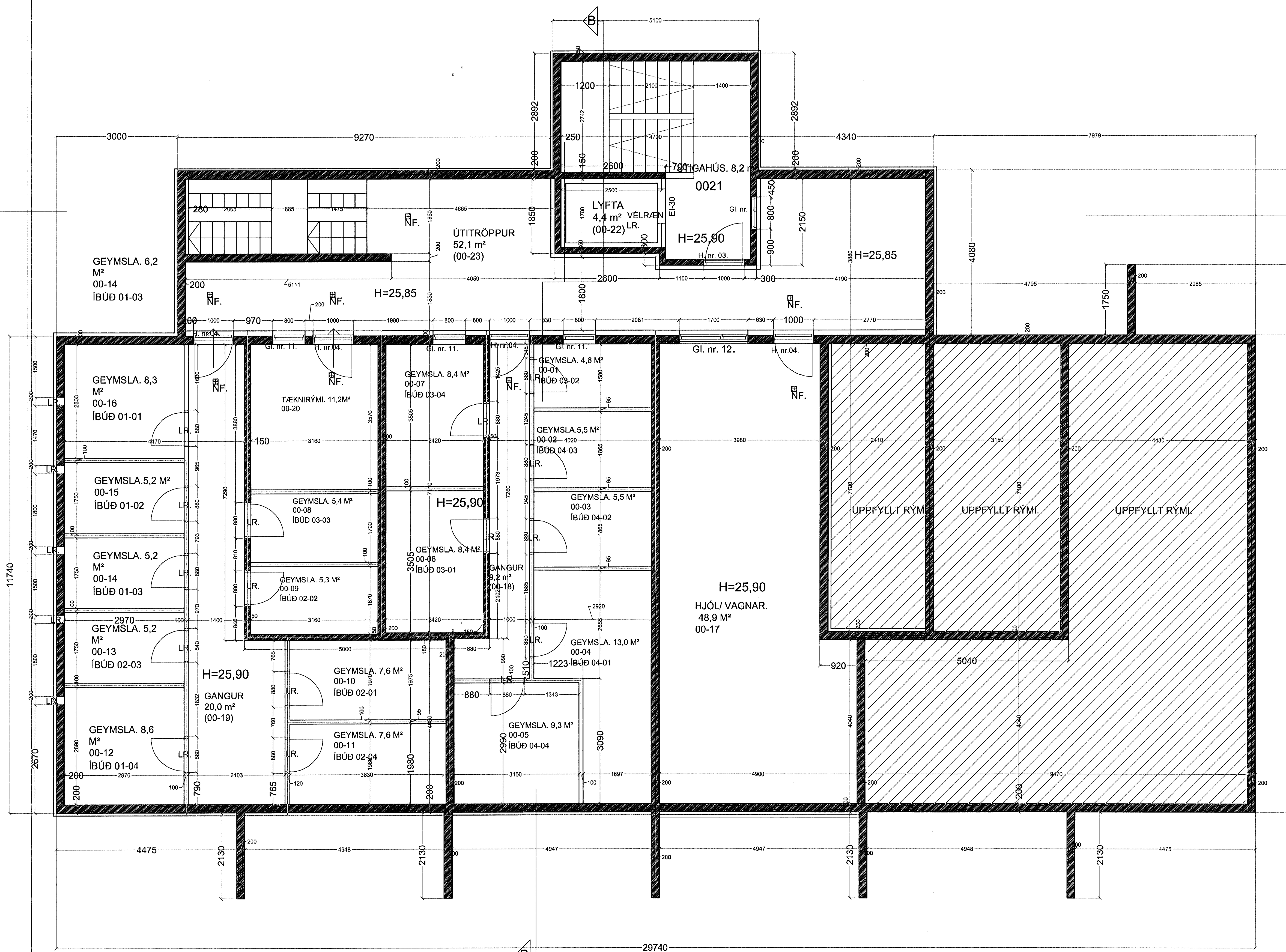
GRUNNMYND KJALLARA. MKV. 1:50.
