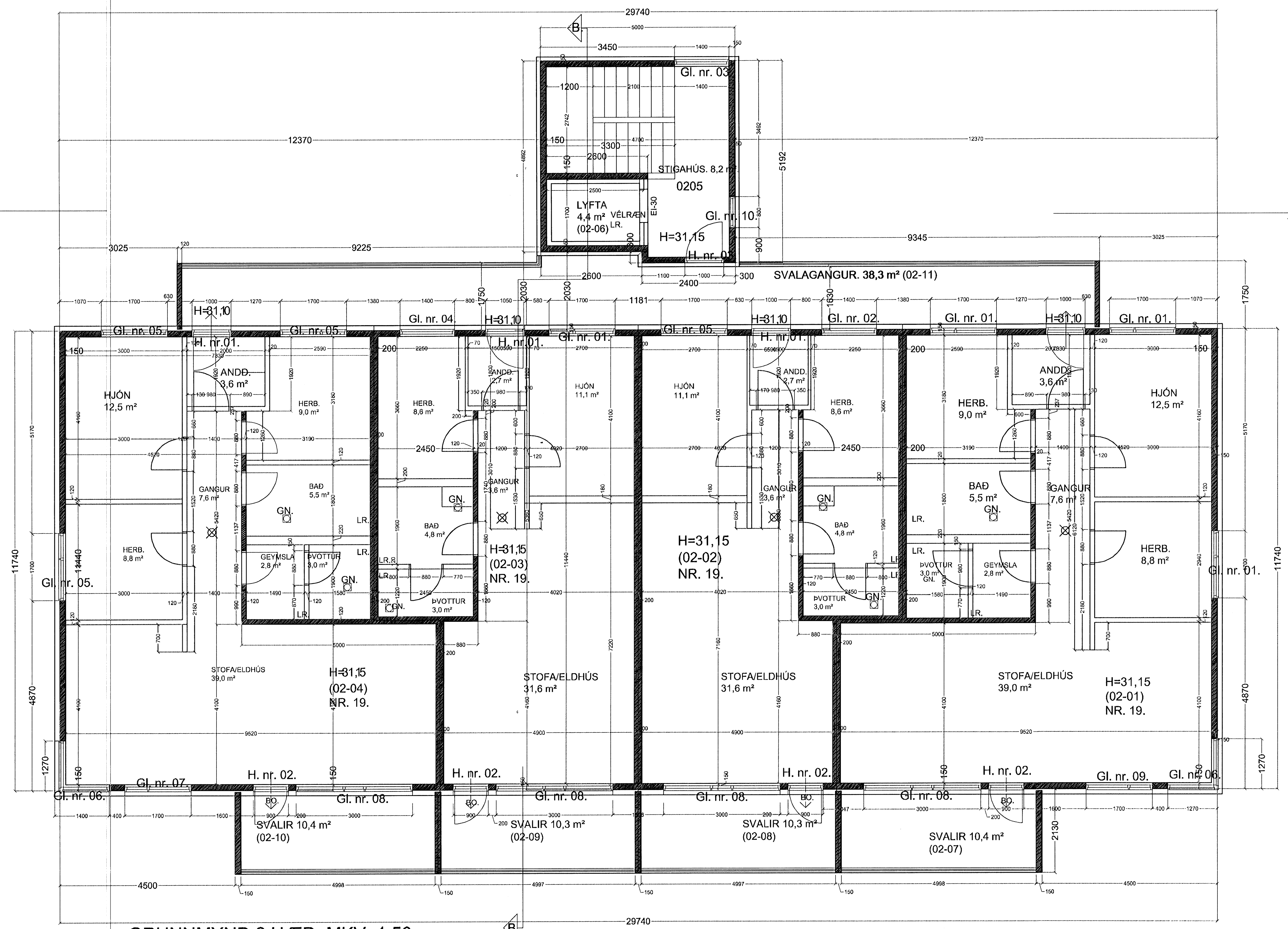
GRUNNMYND 2 HÆÐ. MKV. 1:50.
