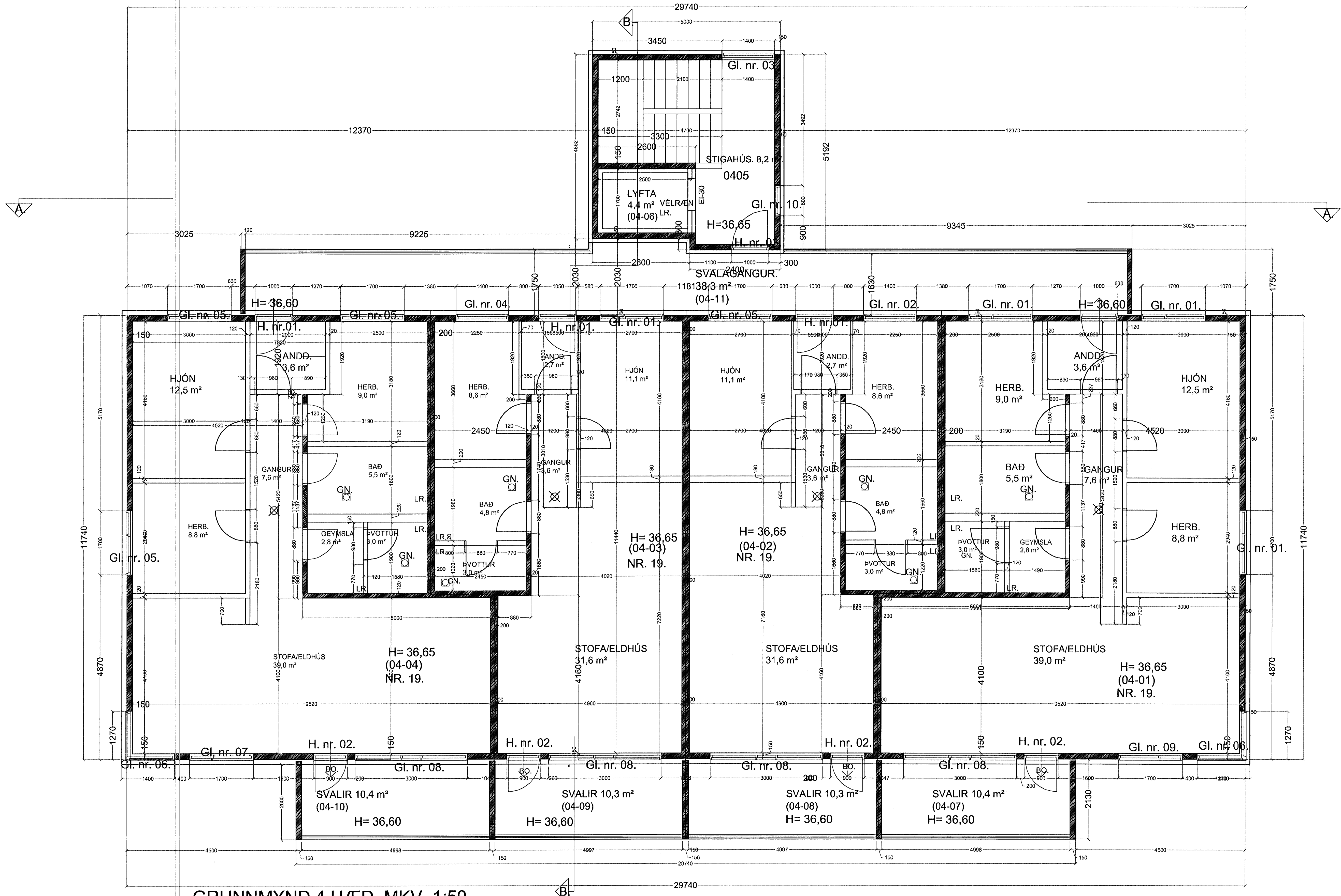
GRUNNMYND 4 HÆÐ. MKV. 1:50.
