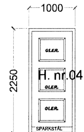
ÚTIDYRAHURÐIR KJALLARA. 2 STK HURÐ OPNIST INN V. 2 STK HURÐ OPNIST INN H.
