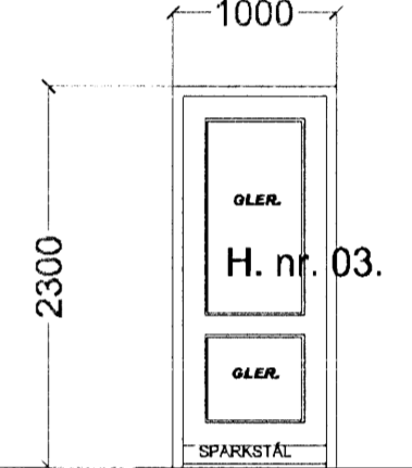
ÚTIDYRAHURÐIR STIGAHÚS 5 STK HURÐ OPNIST INN V.
