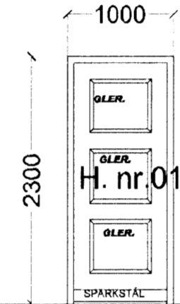
ÚTIDYRAHURÐIR 8 STK HURÐ OPNIST INN V. 8 STK HURÐ OPNIST INN H.
