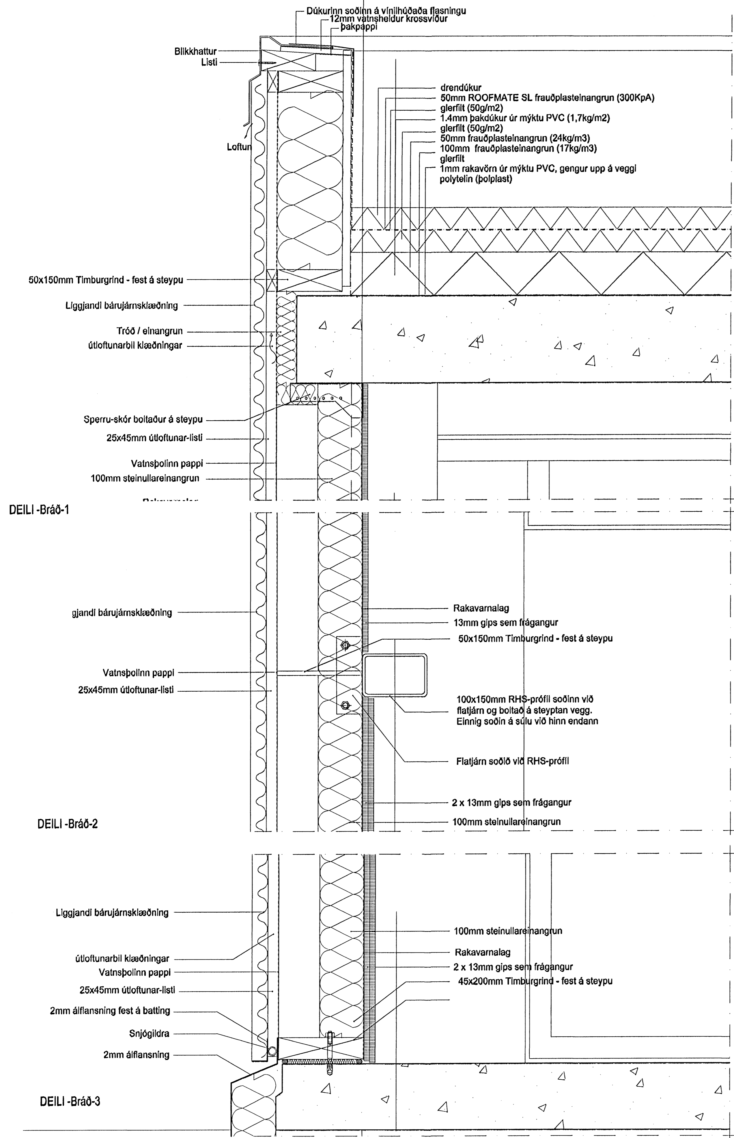
FRÁGANGUR BRÁÐAGRIGÐAVEGGJAR - LÓDRÉTT SNIÐ MKV. 1:5
