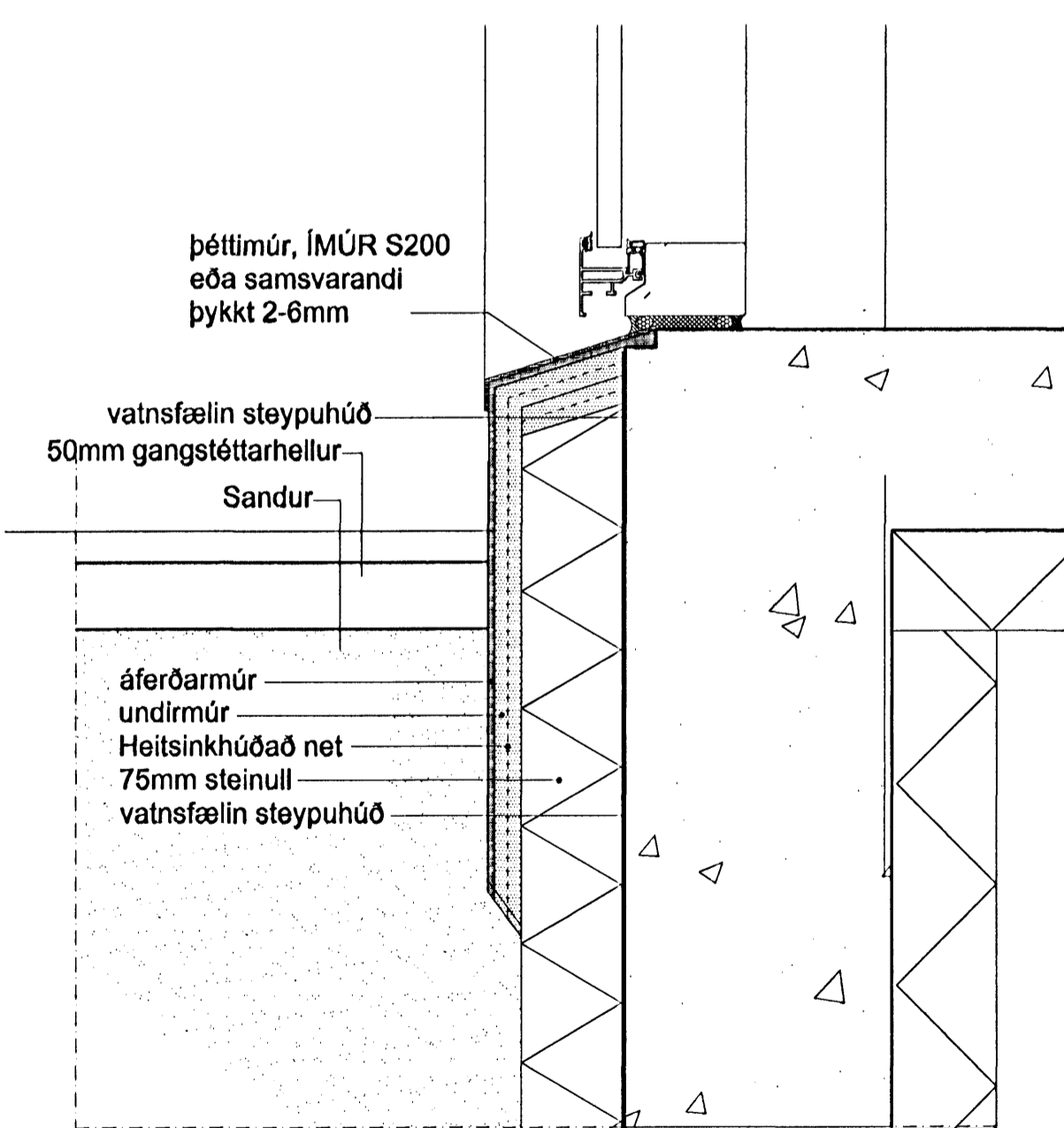
FRÁGANGUR GÓLFSÍÐRA GLUGGA
