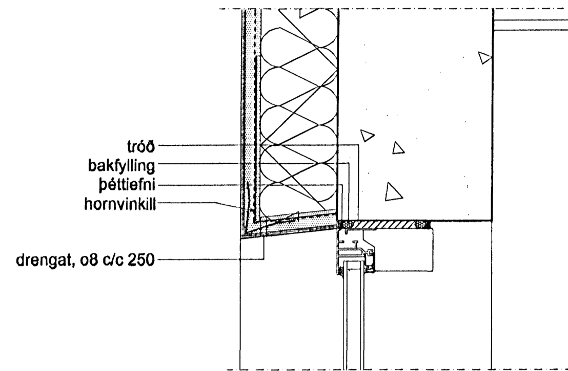
FRÁGANGUR ÍMÚRKLÆDNINGAR OFAN VÍÐ GLUGGA
