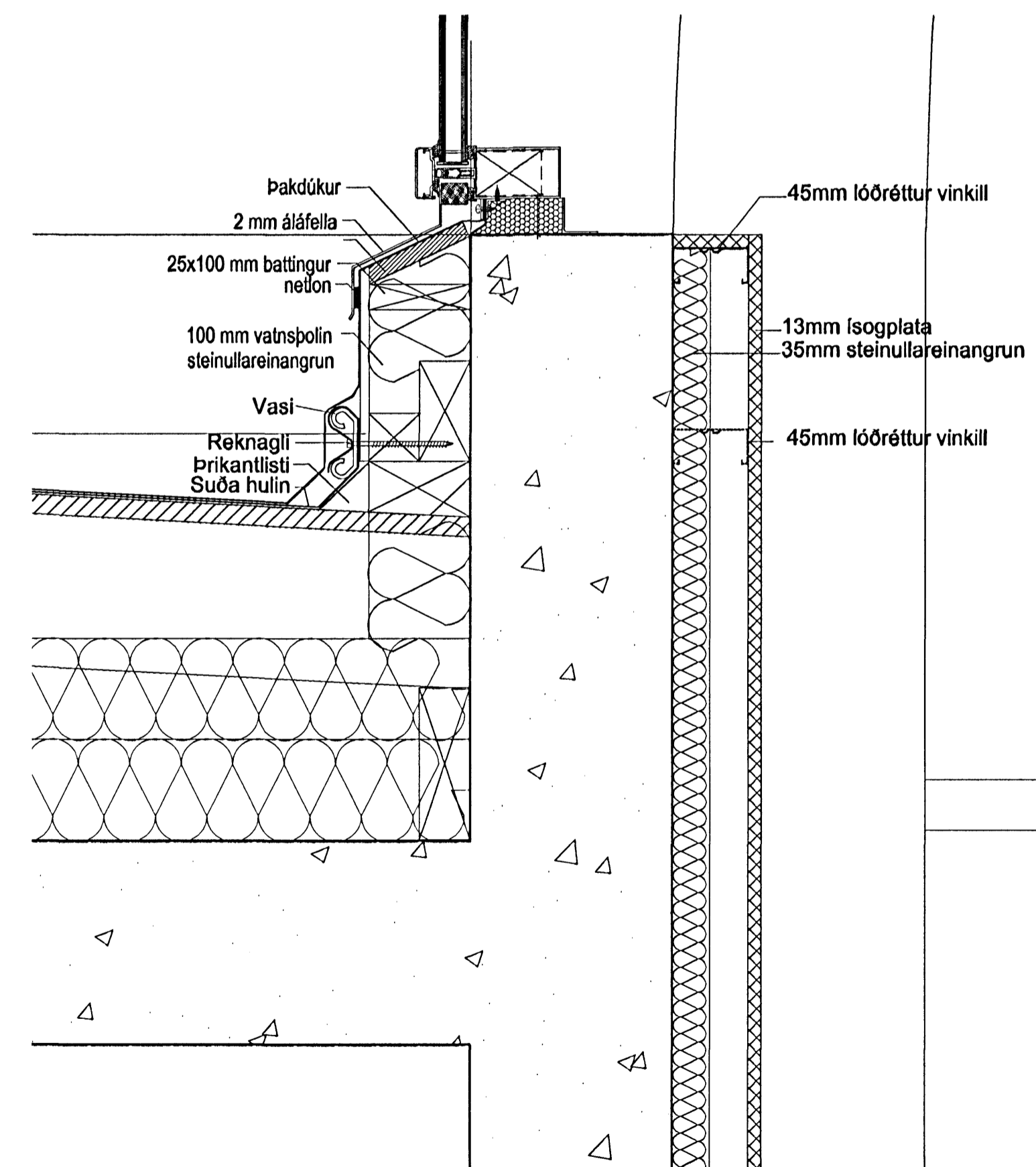
FRÁGANGUR GLERVEGGJAR OFAN Á HÚSI A
