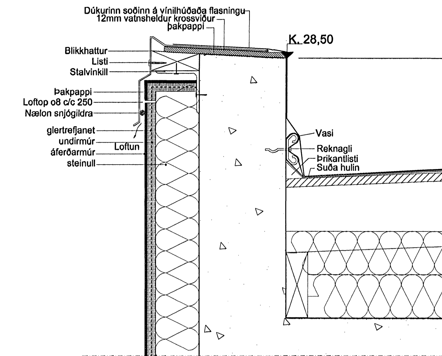
FRÁGANGUR ÞAKS OG ÞAKKANTA ÍMÚRKLÆDDIR VEGGIR
