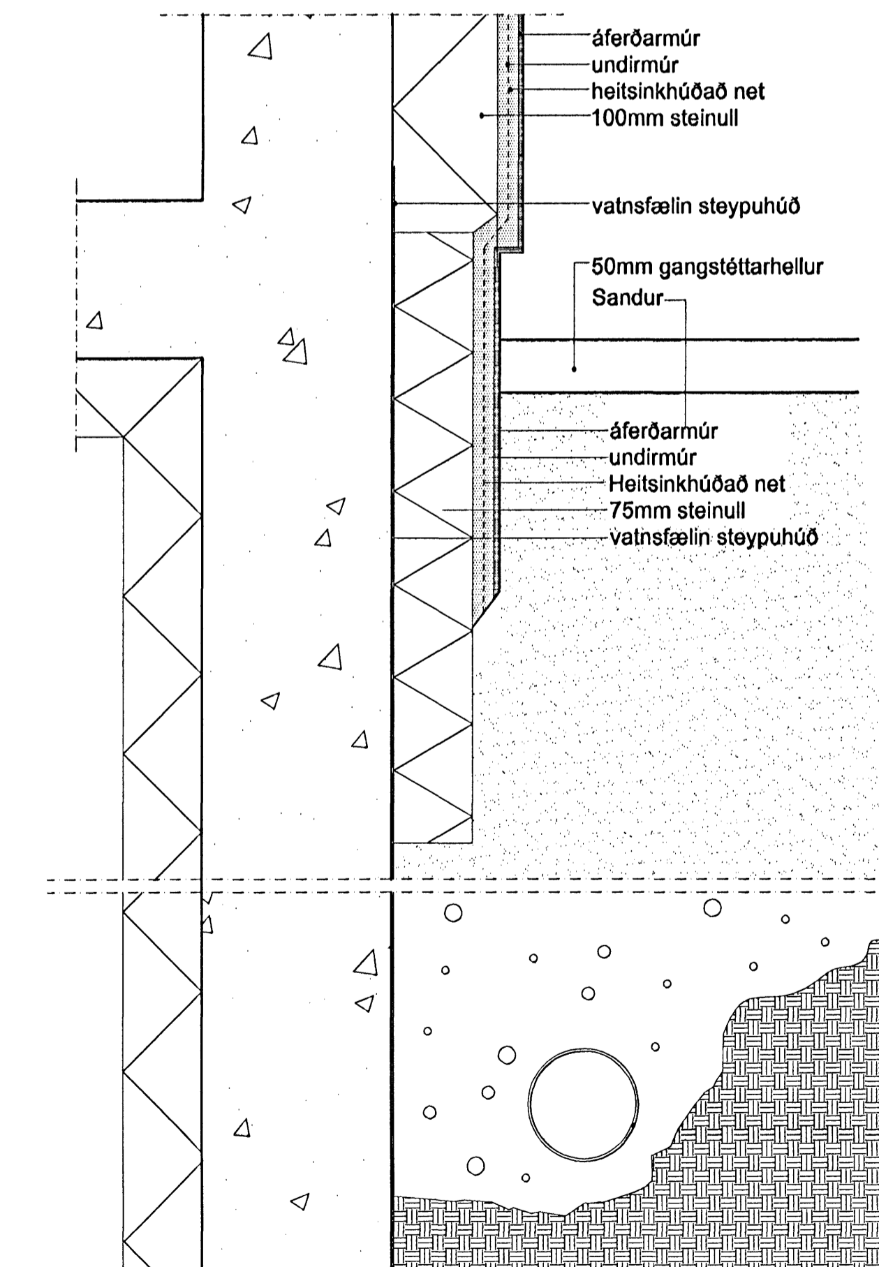
FRÁGANGUR ÍMÚRKLÆDDRA VEGGJA VÍÐ JÖRD
