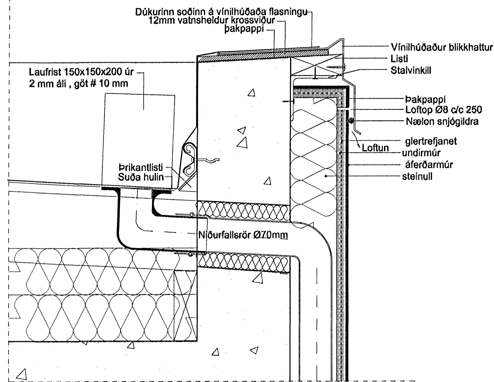
FRÁGANGUR ÞAKS OG ÞAKKANTA VÍÐ NIÐURFÖLL ÍMÚRKLÆDDIR VEGGIR
