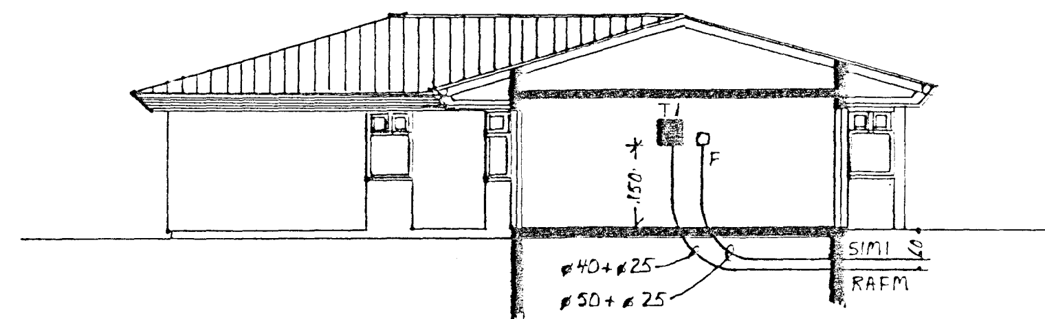
SNEIÐING M 1:100
