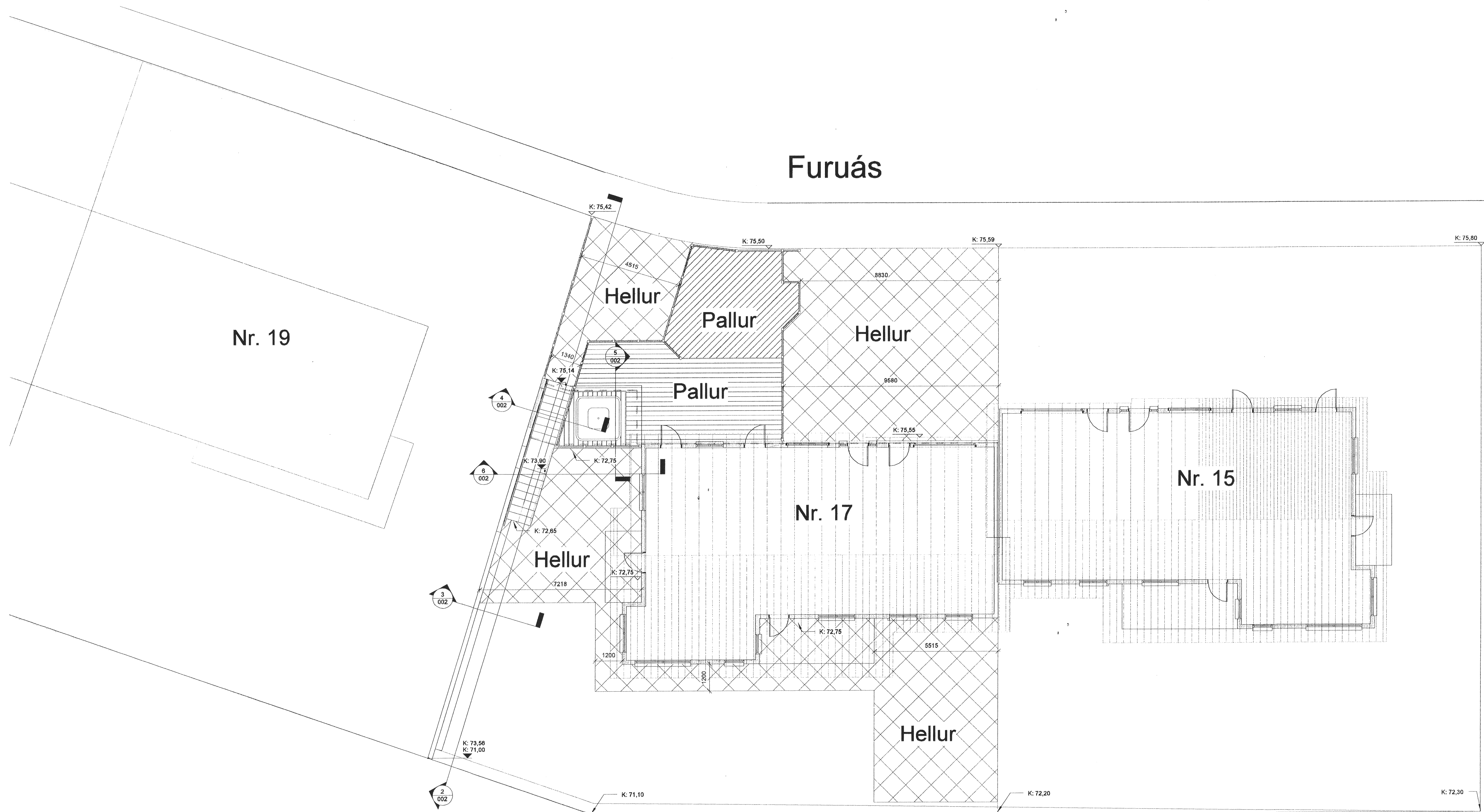
1 Grunnmynd 1 : 100
