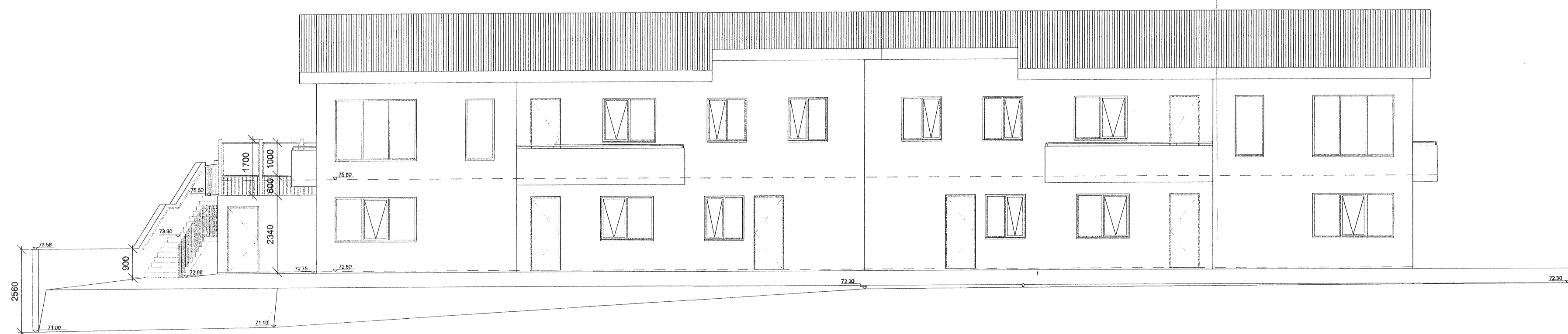
2 Norður útlit 1 : 100
