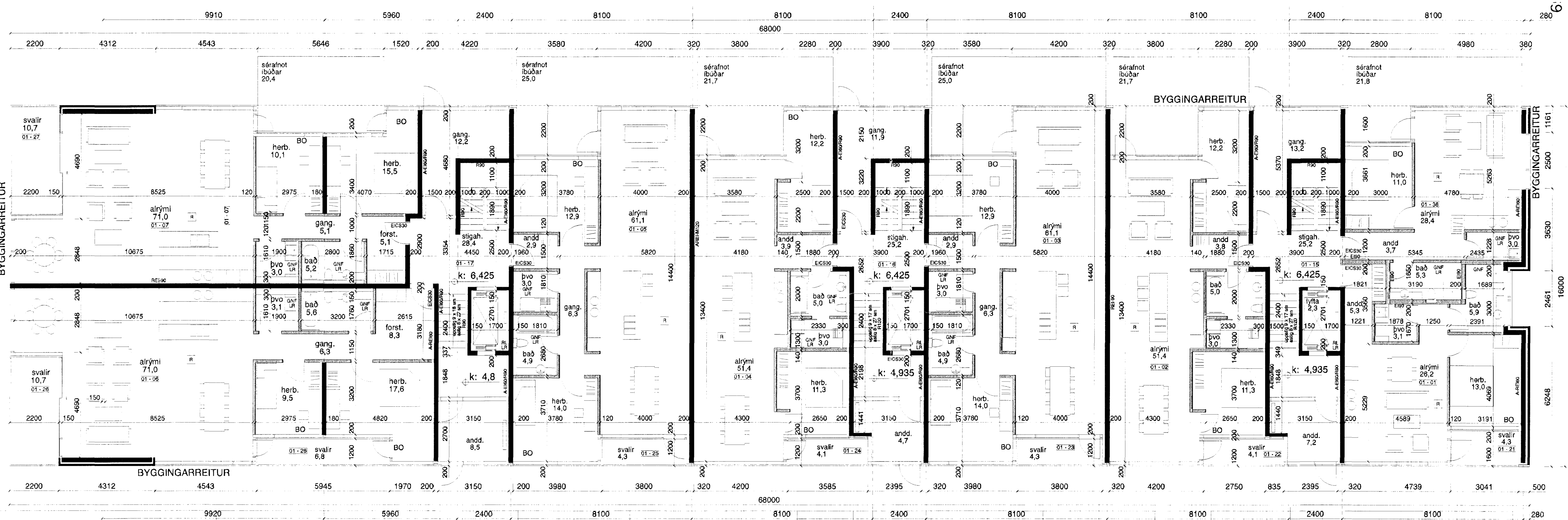
Norðurbakki 9 jarðhæð 1:100
