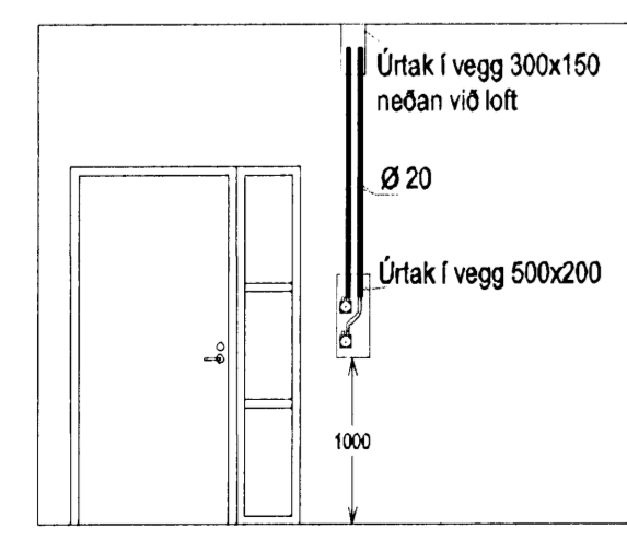
Dæmi um frágang þar sem fleiri en 1 dós eru sýndar
