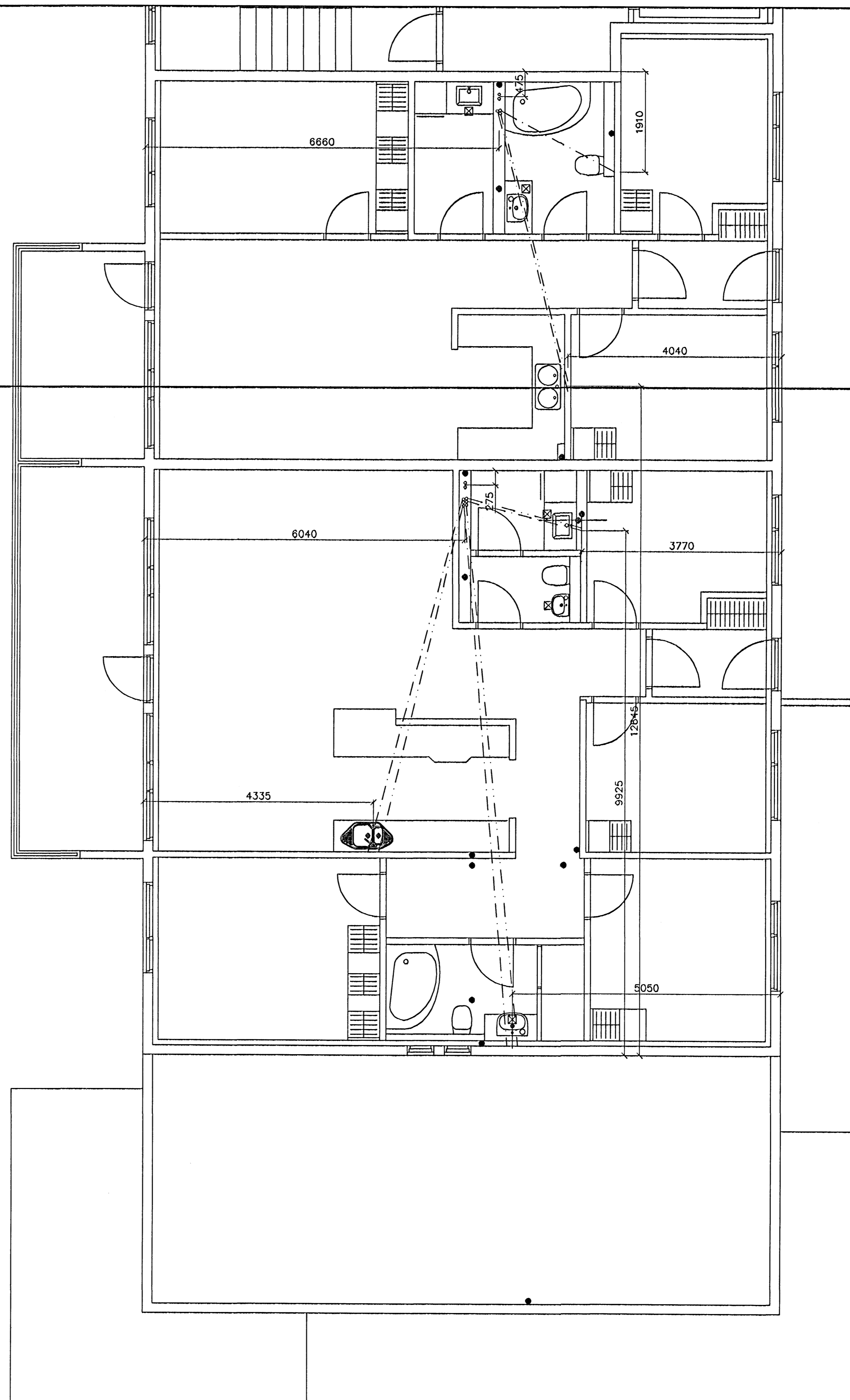
GRUNNMYND 4 HÆÐAR 1:50
