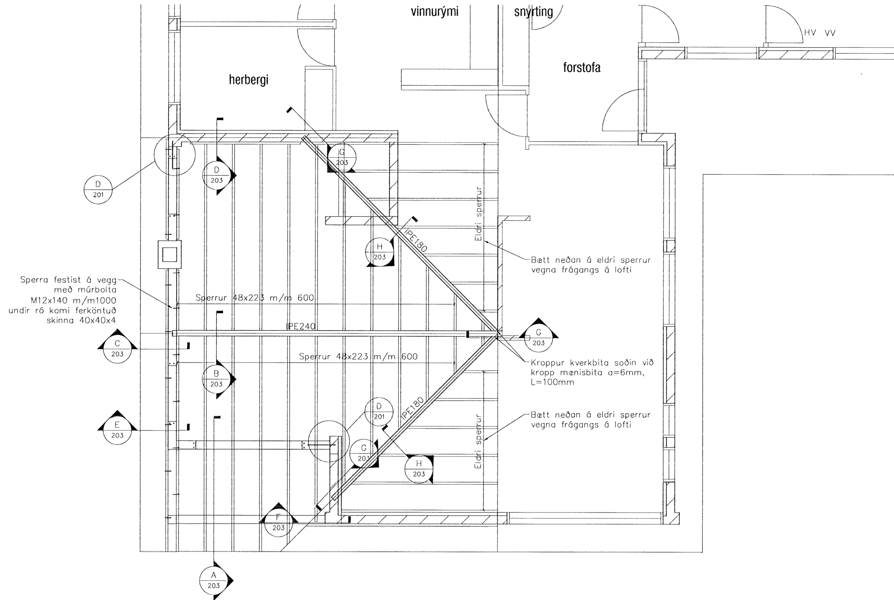
Grunnmynd 1 = 50 mm
