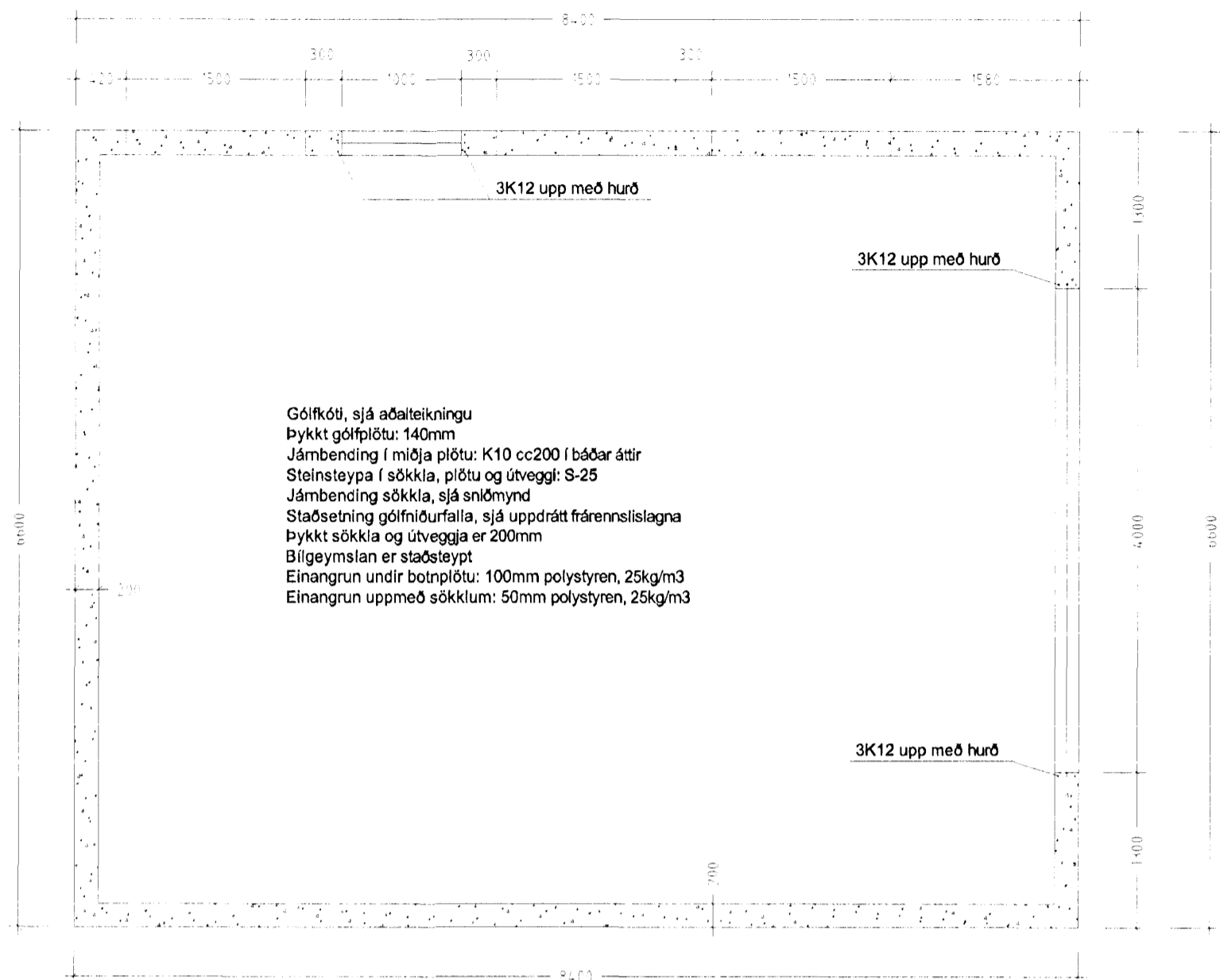
Grunnmynd sókkla Mkv.1/50
