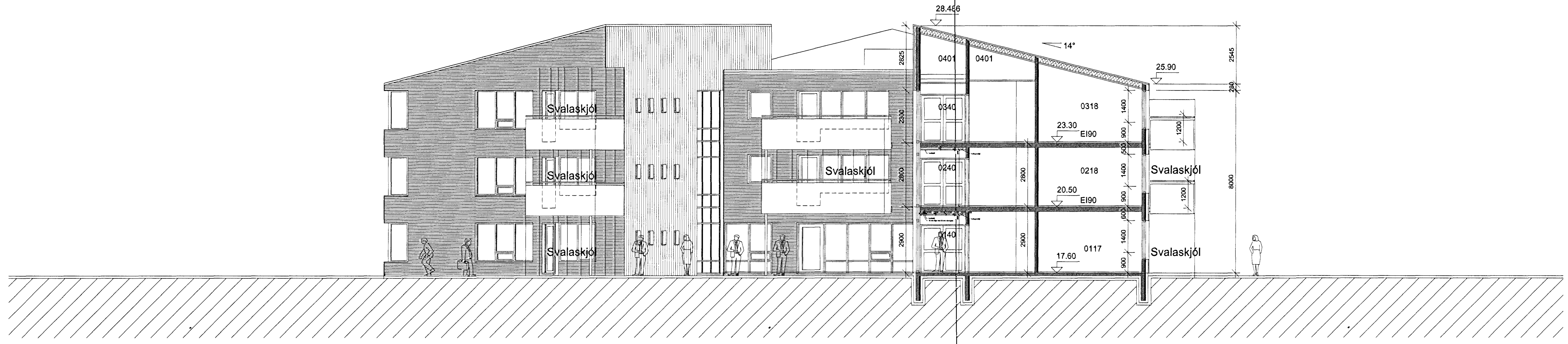
HRAUNVANGUR 3 SNÍÐ F-F 1:100
