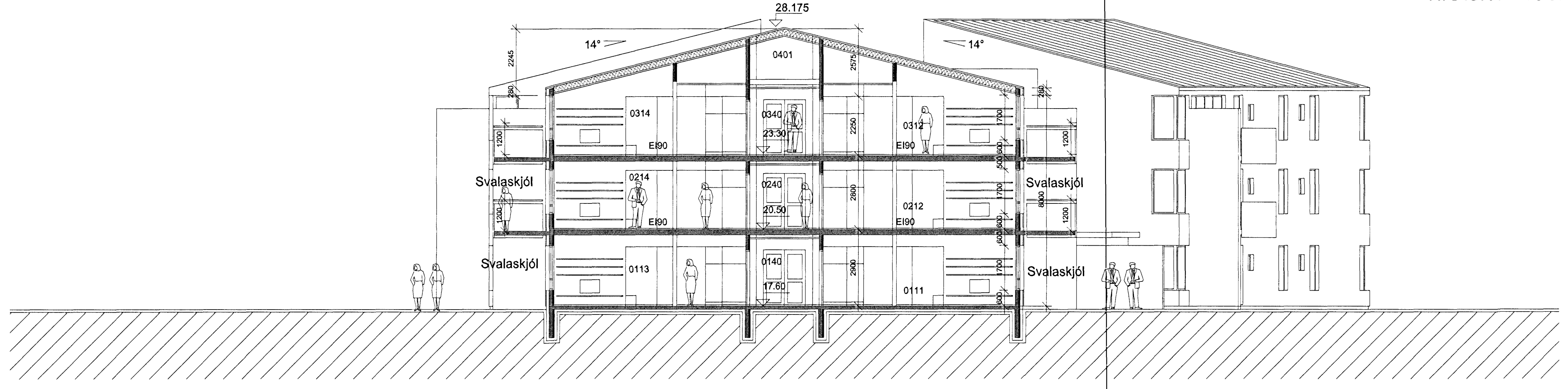
HRAUNVANGUR 3 SNÍÐ D-D 1:100
