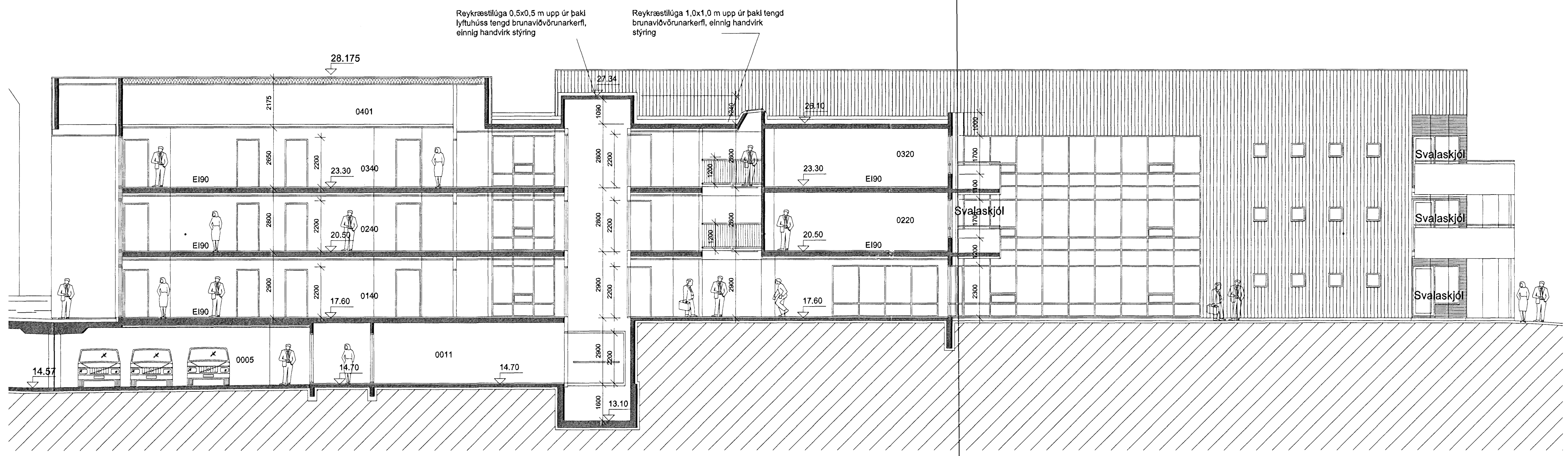
HRAUNVANGUR 3 SNÍÐ E-E 1:100
