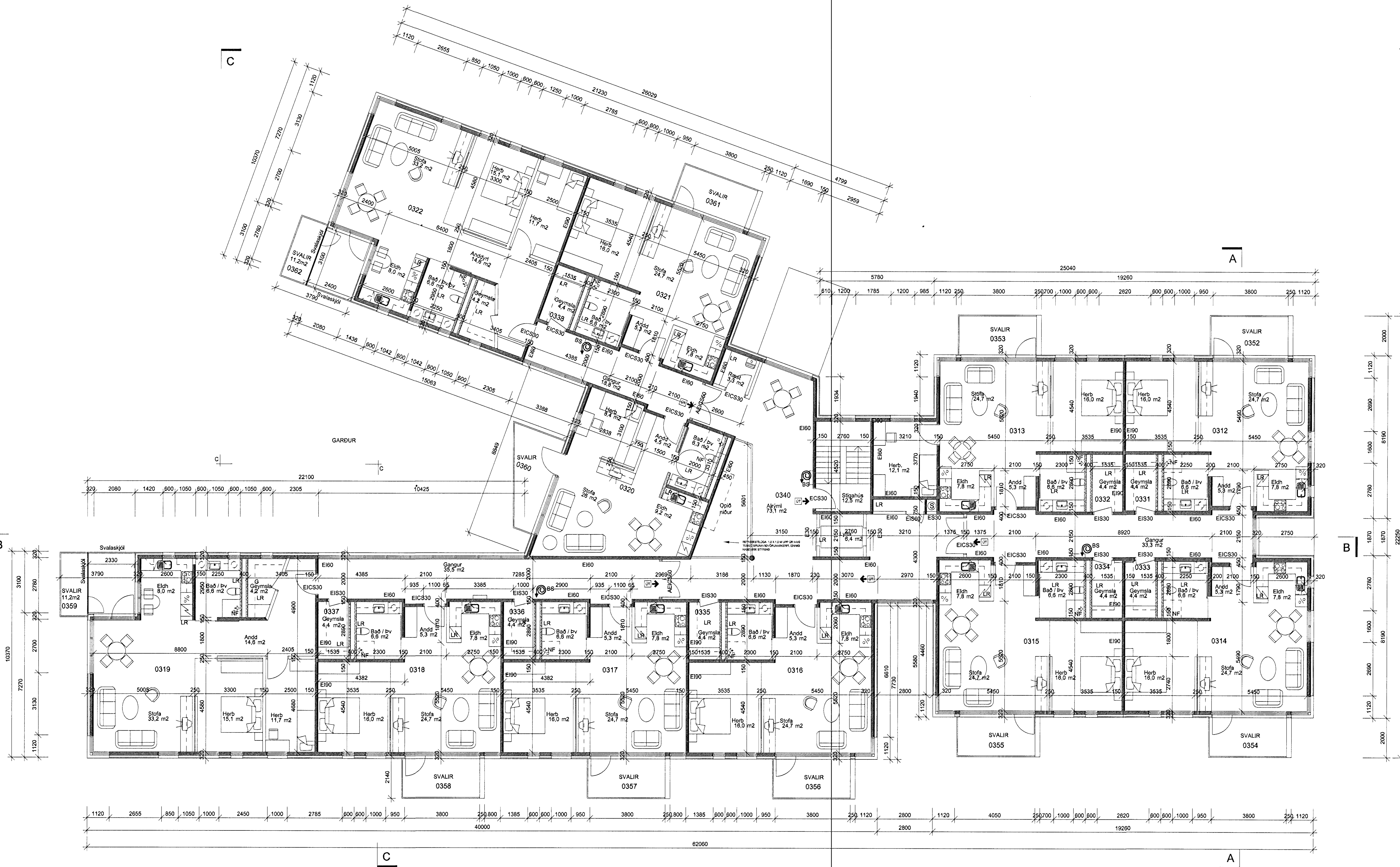
GRUNNMYND 3.HÆÐ 1:100
