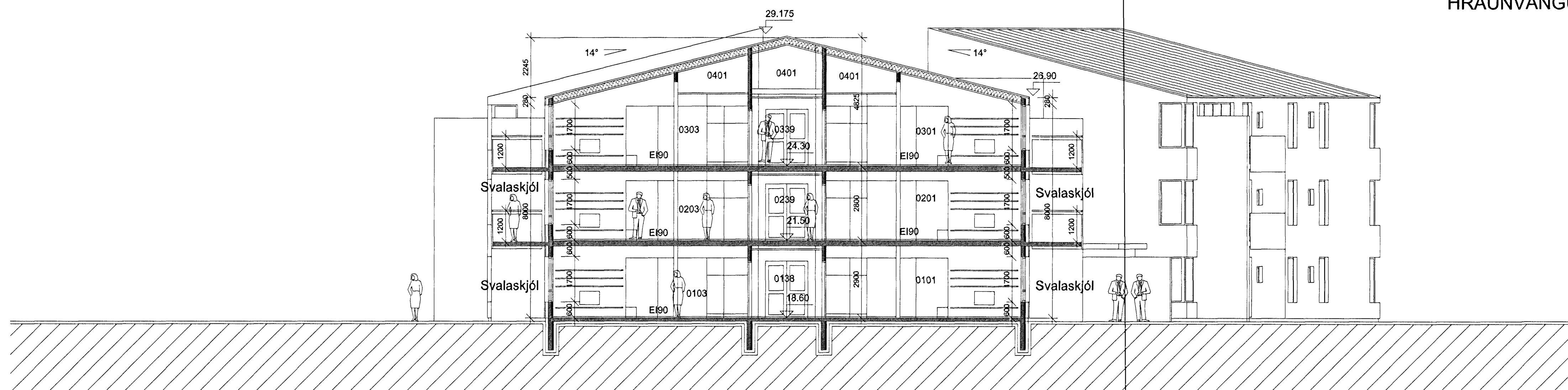
HRAUNVANGUR 1 SNID A-A 1:100
