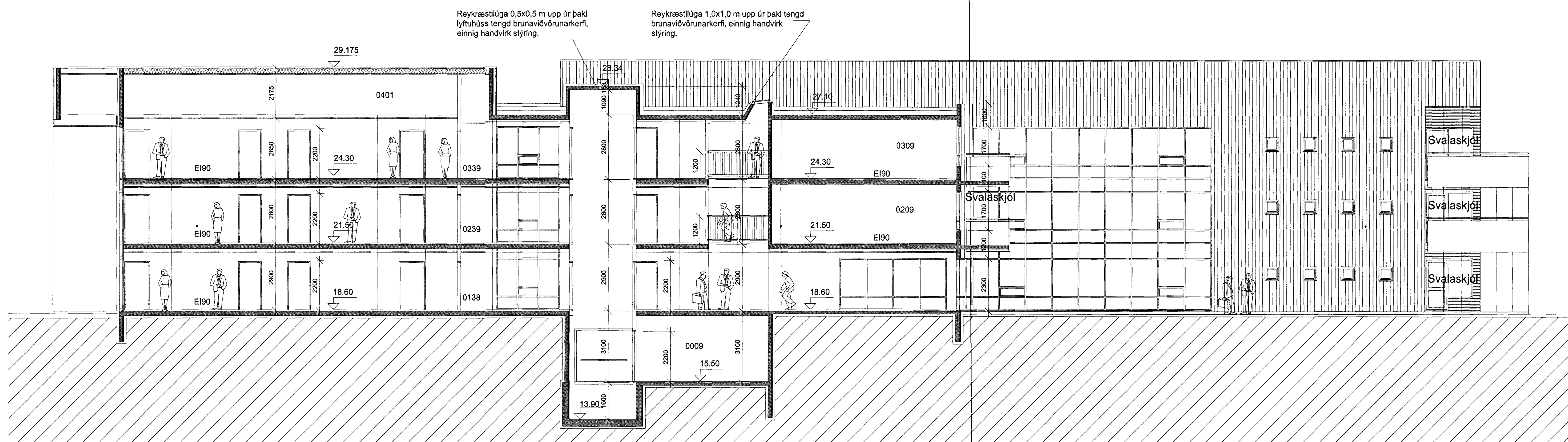
HRAUNVANGUR 1 SNID B-B 1:100
