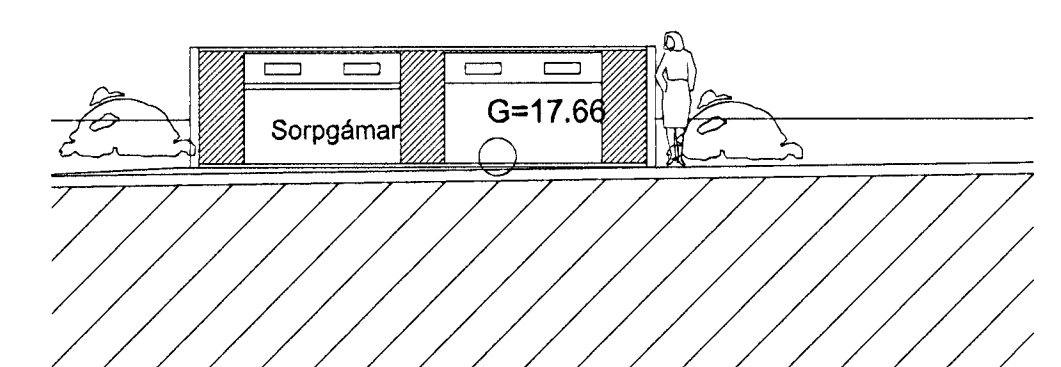
TIMBURGIRÐING UMHVERFIS SORPGÁMA ÚTLIT NORÐUR 1:100
