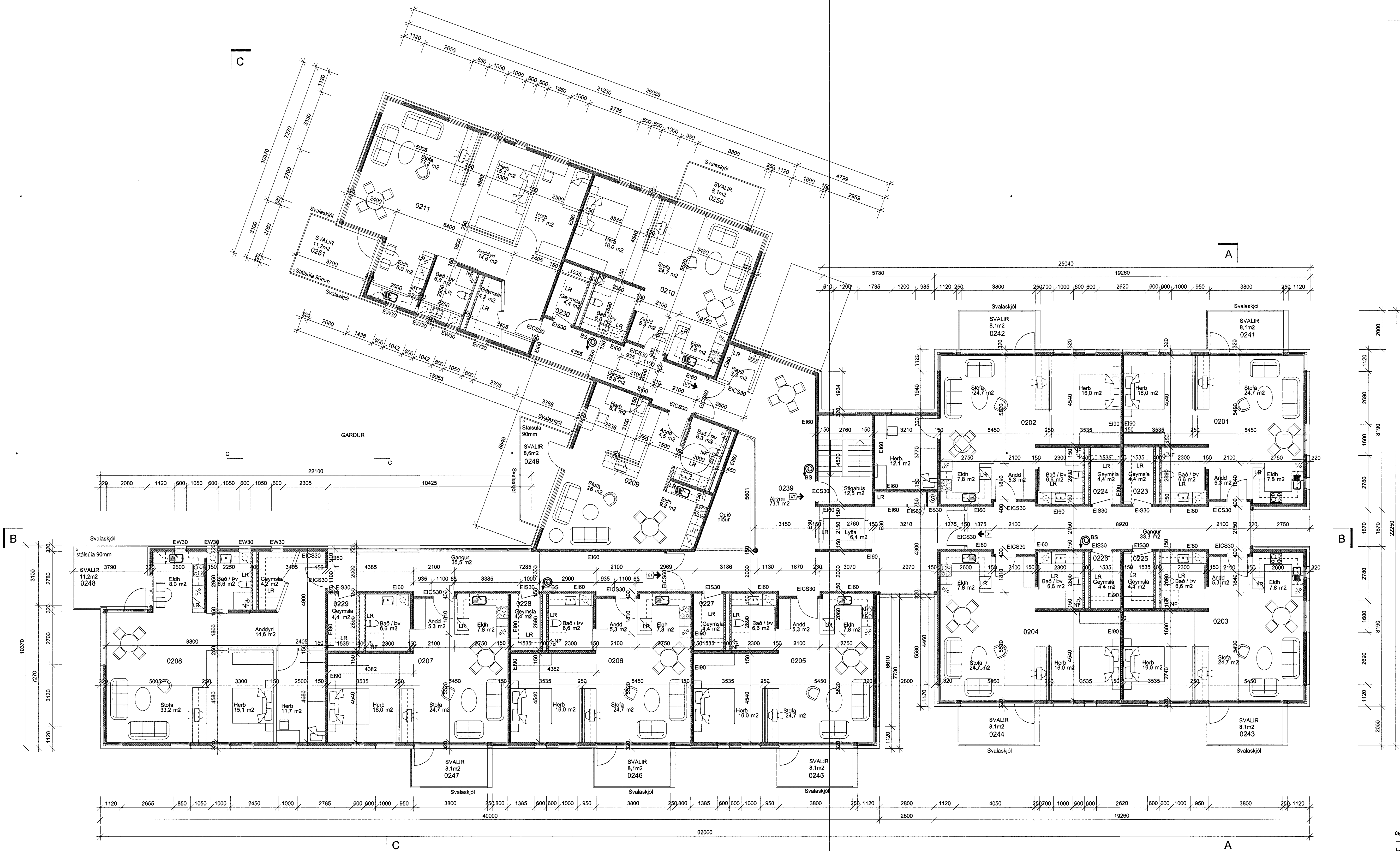
GRUNNMYND 2.HÆÐ 1:100
